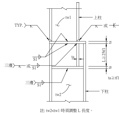
c. H 形柱偏心
