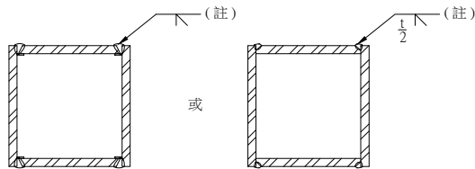
d.組合箱形
