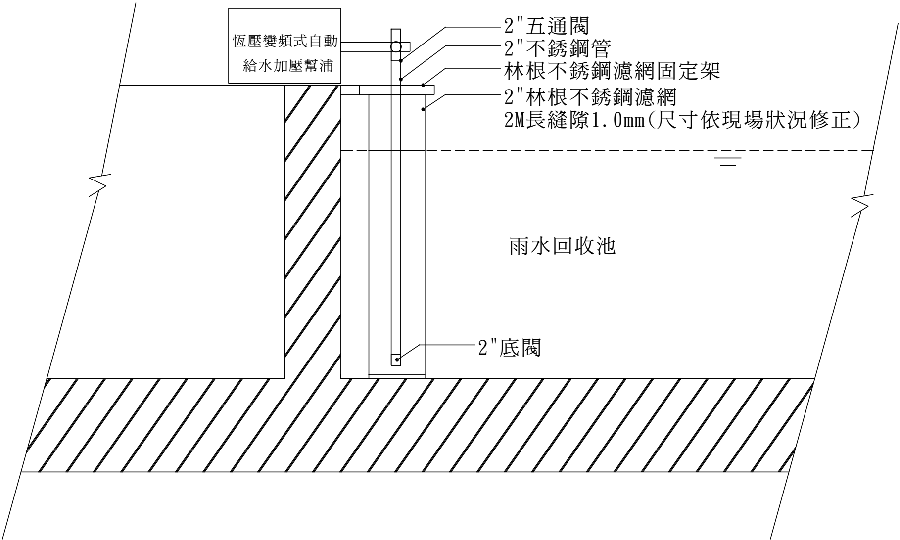
1 噴灌單線圖
