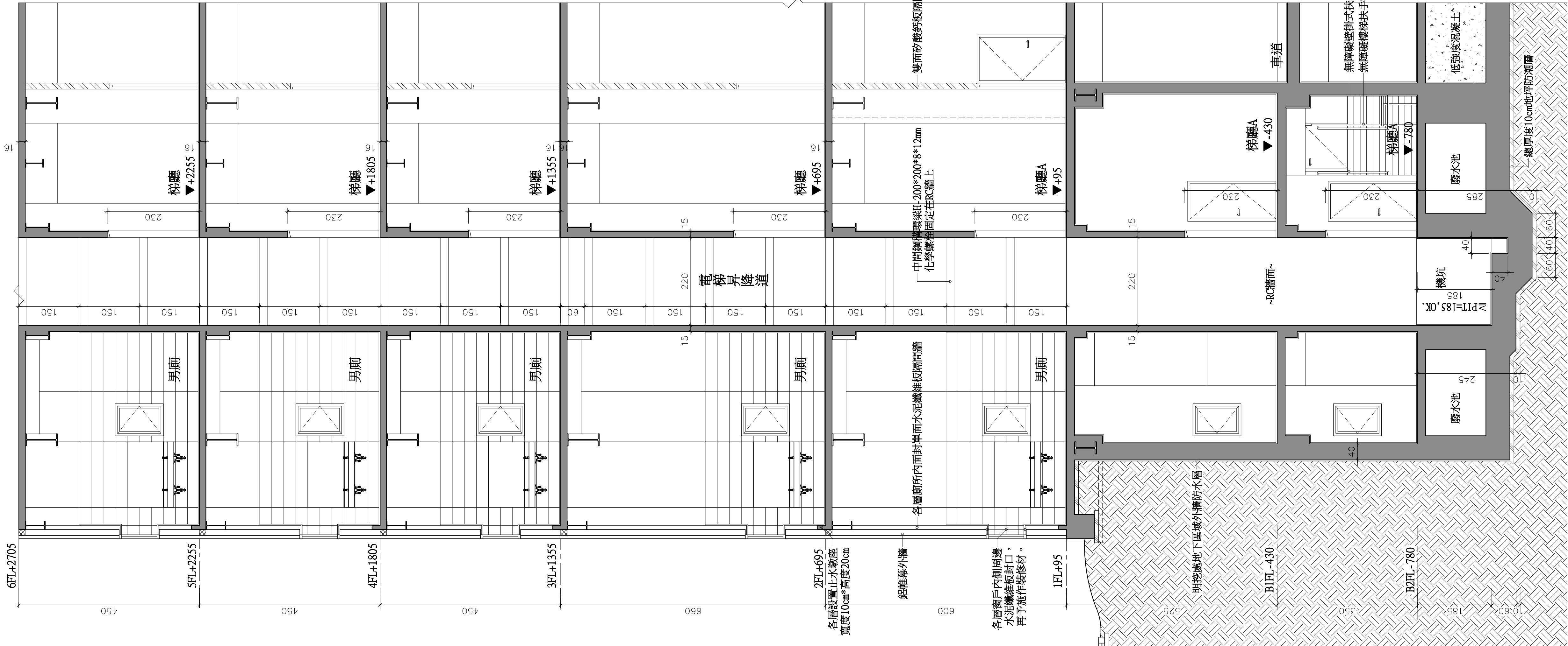
1/ A4-7 NO.1 電梯升降道及廁所剖面圖(一) A1=S:1/60 A3=S:1/120
