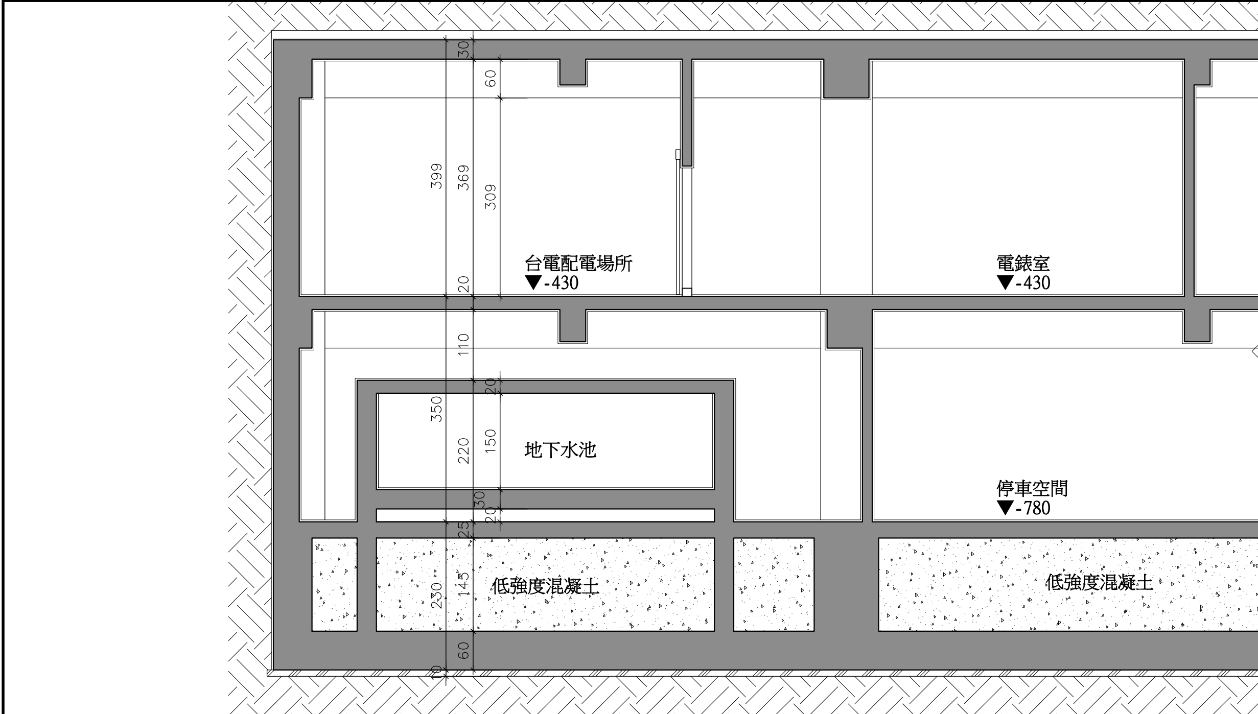
2 A4-6 外牆剖面圖 A1=S:1/60 A3=S:1/120
