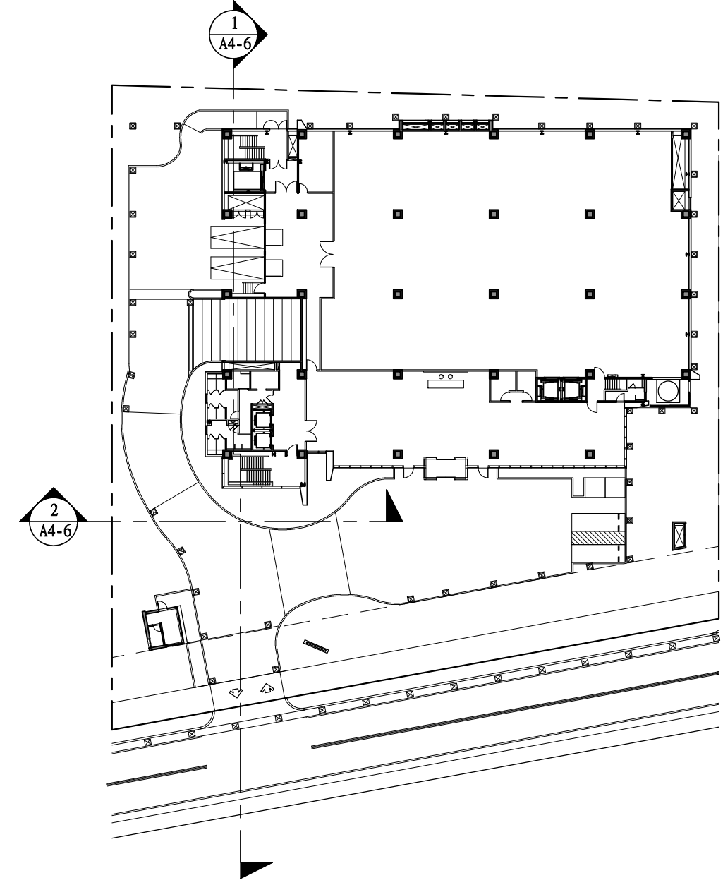
3 A4-6 剖面索引圖
