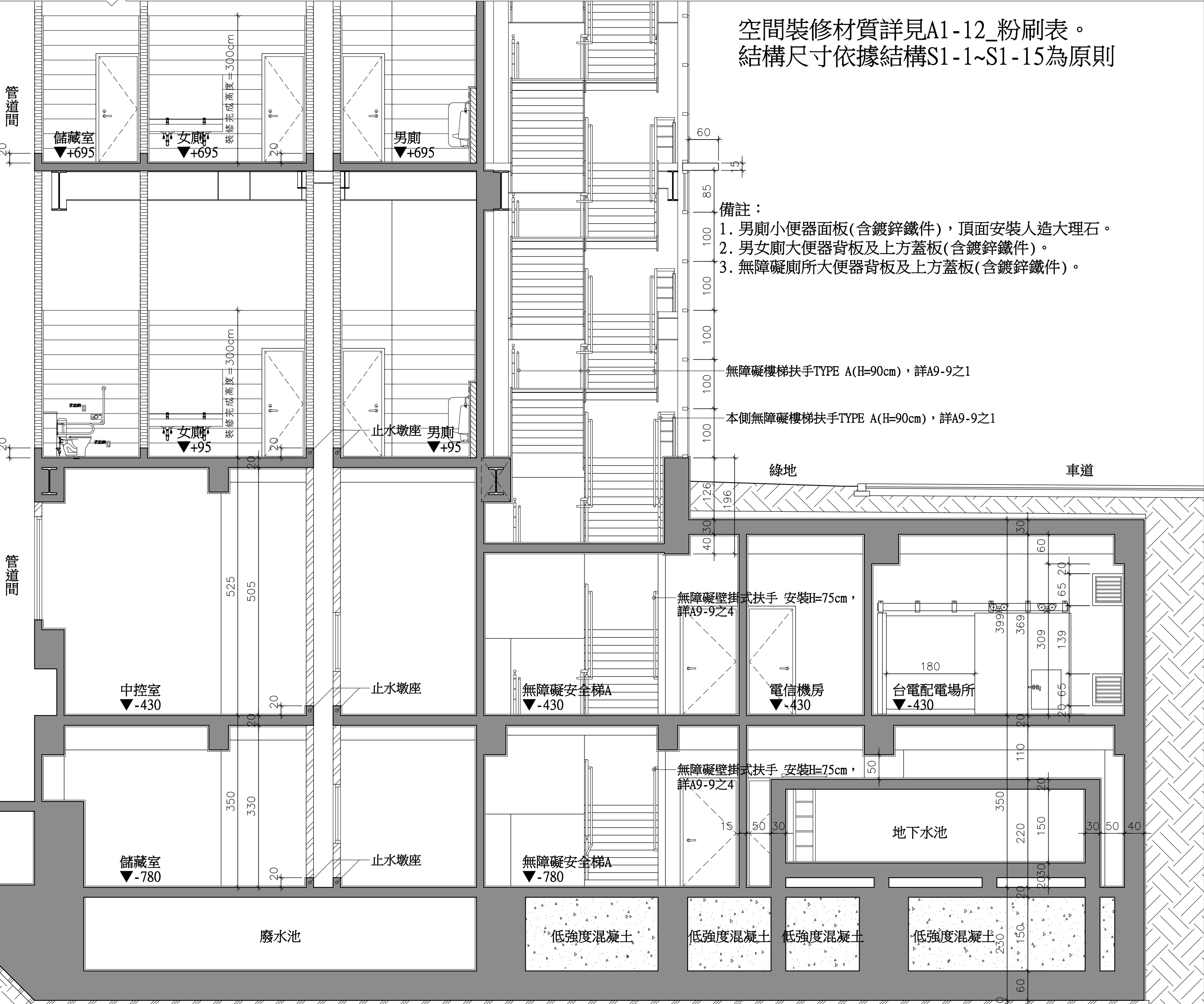
3 A4-6 剖面索引圖
