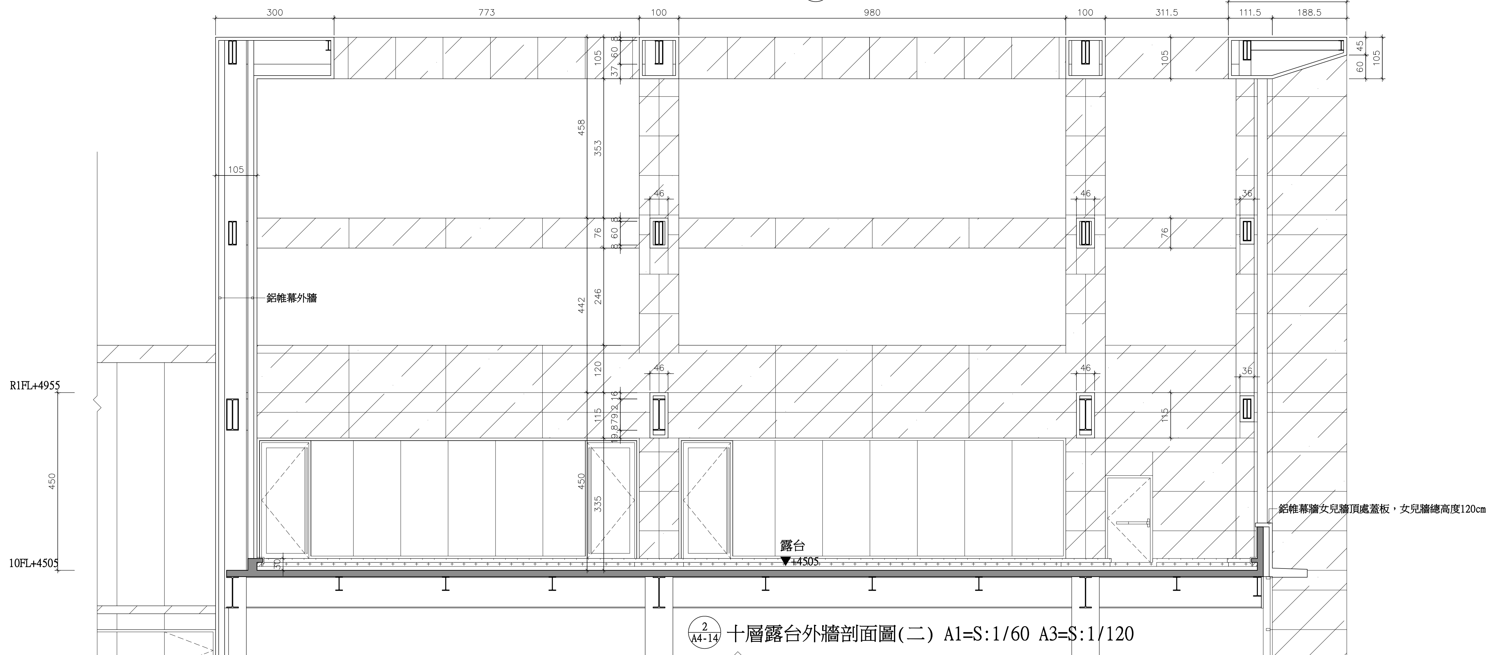
1 十層露台外牆剖面圖(一) A1=S:1/60 A3=S:1/120
