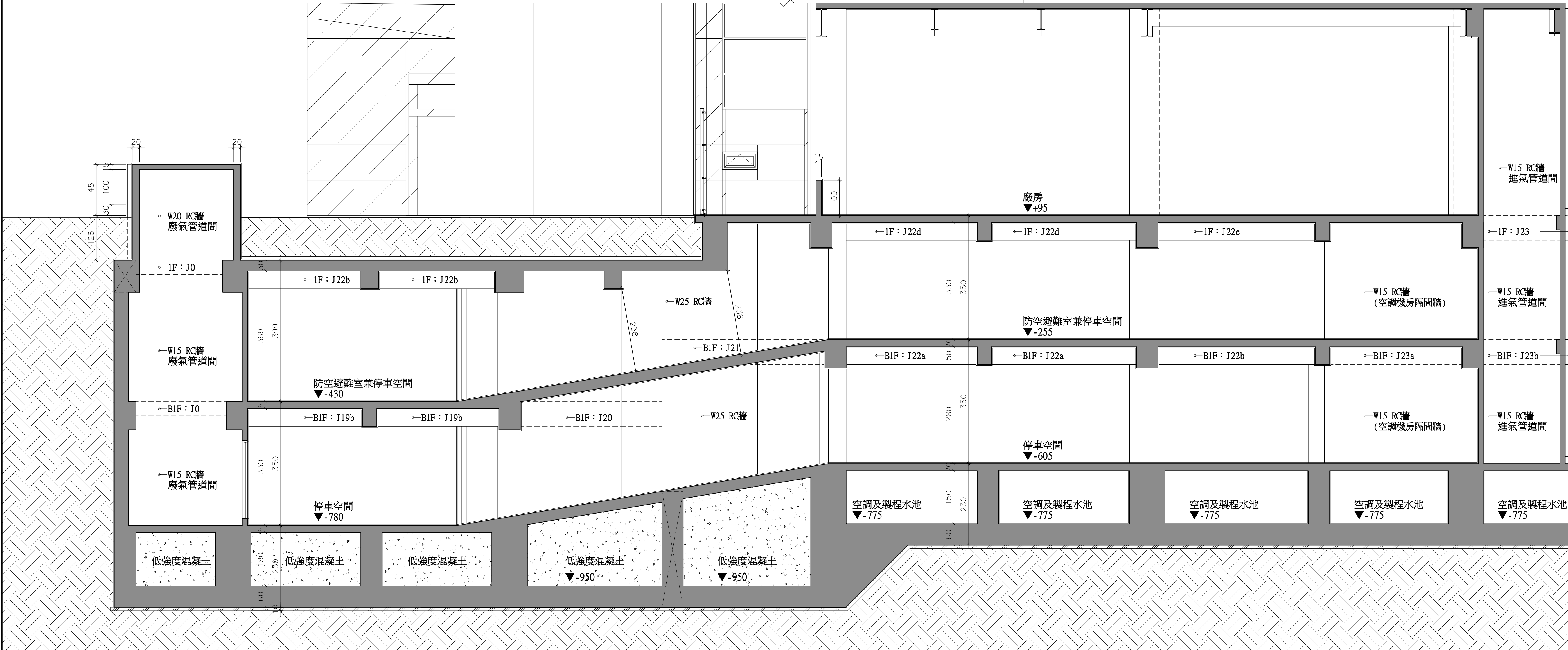
LINE5~6 地下層車道及外牆剖面圖 A1=S:1/60 A3=S:1/120
