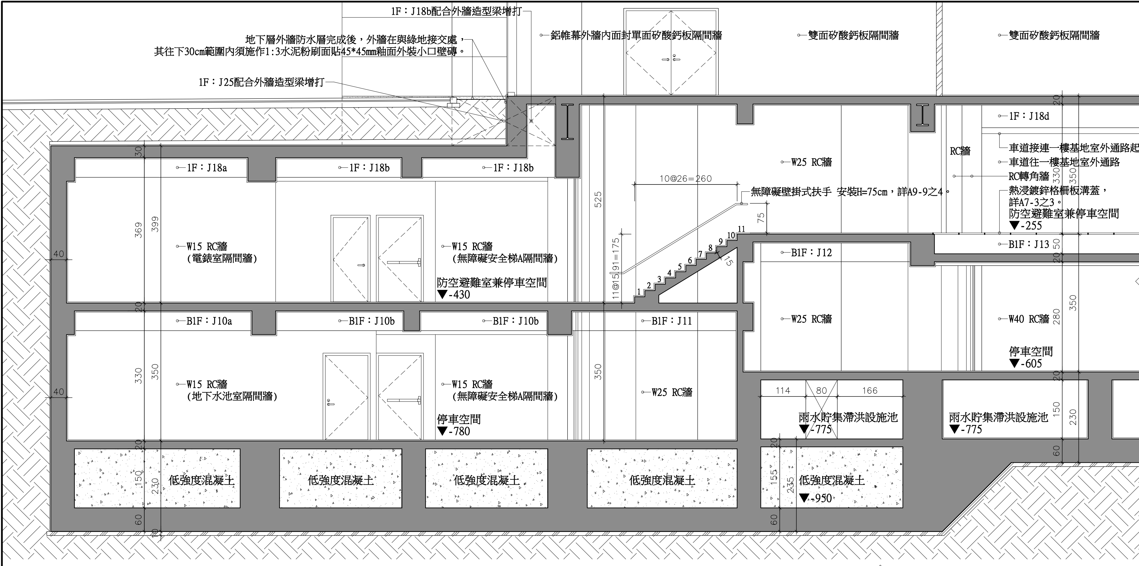
LINE2~3 地下層樓梯及外牆剖面圖 A1=S:1/60 A3=S:1/120
