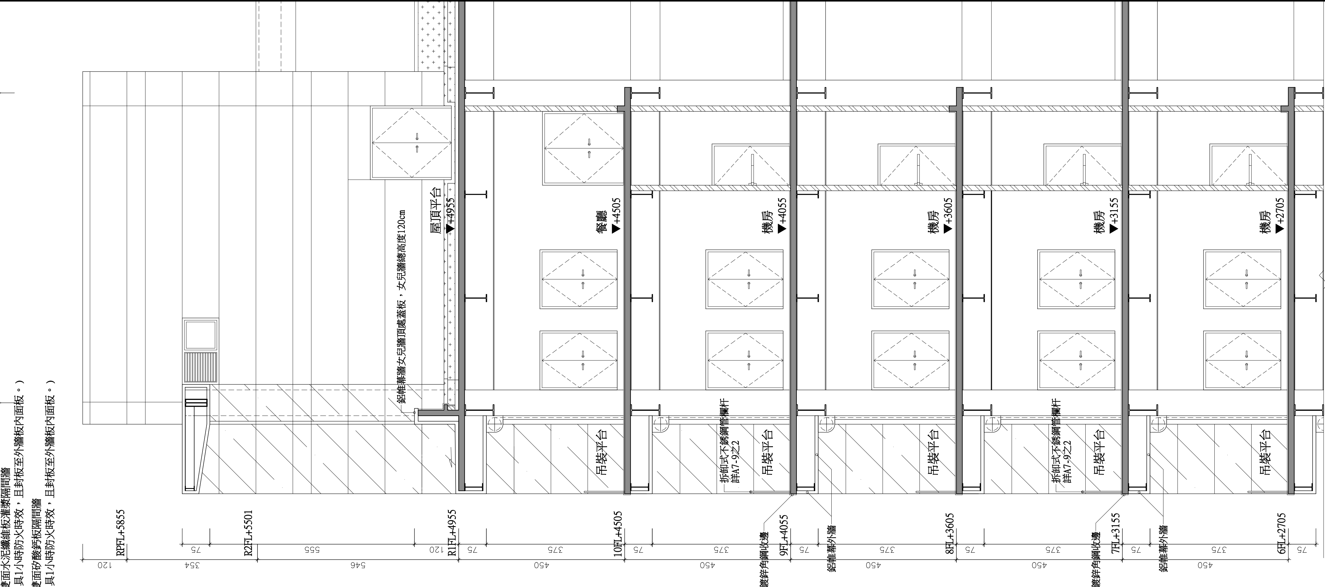
2/44-10 裝卸區外牆剖面圖(二) A1=S:1/60 A3=S:1/120
