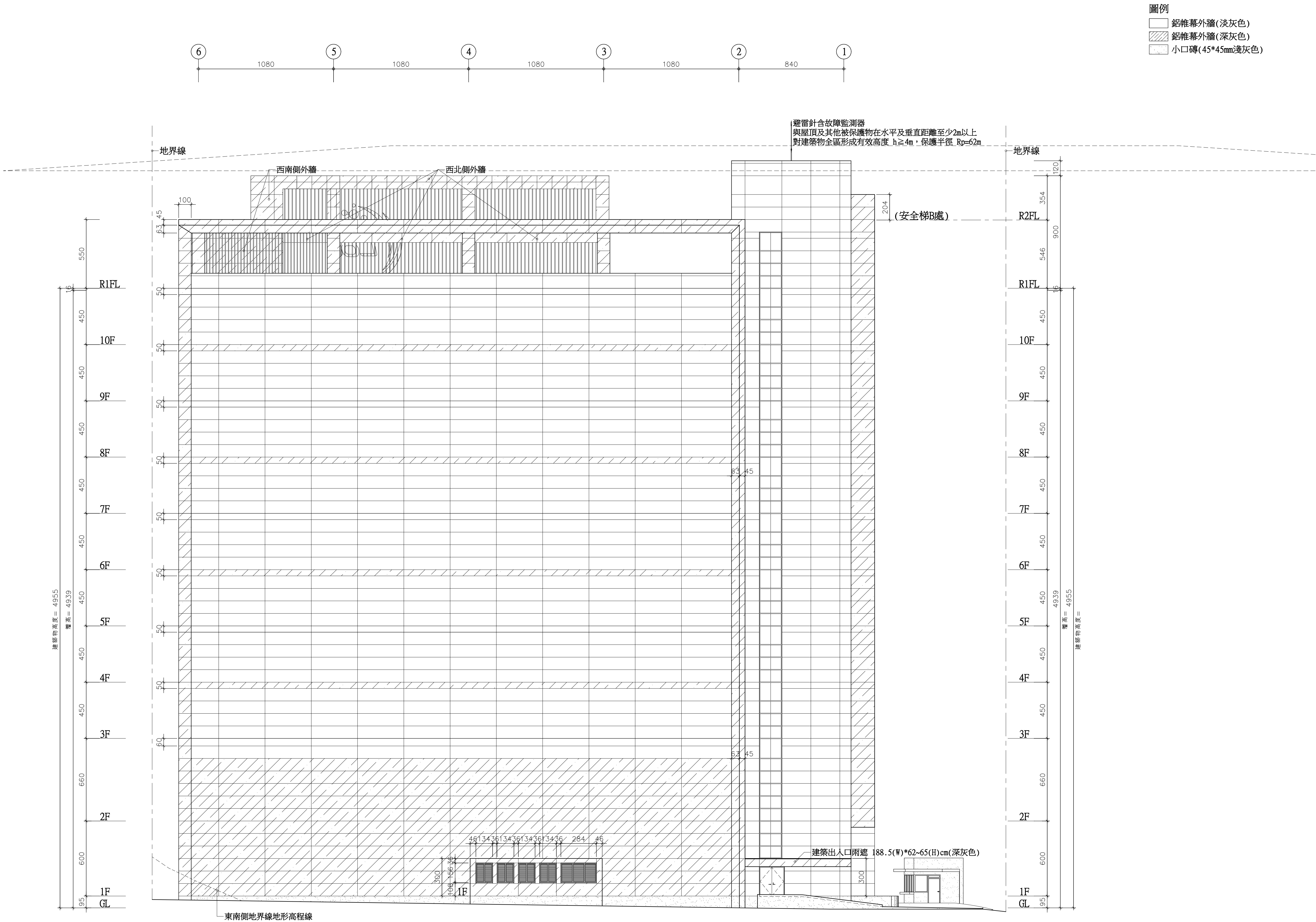
1 A3-2 東南向立面圖 A1=S:1/150 A3=S:1/300
