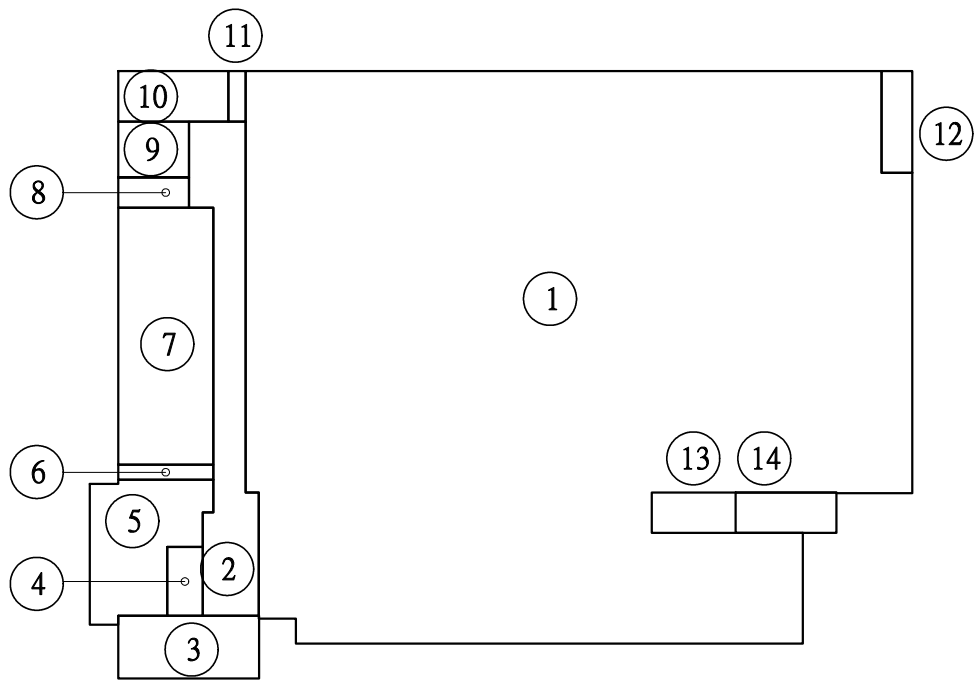
二層防火區劃檢討圖 檢討計算式詳見A1-10
