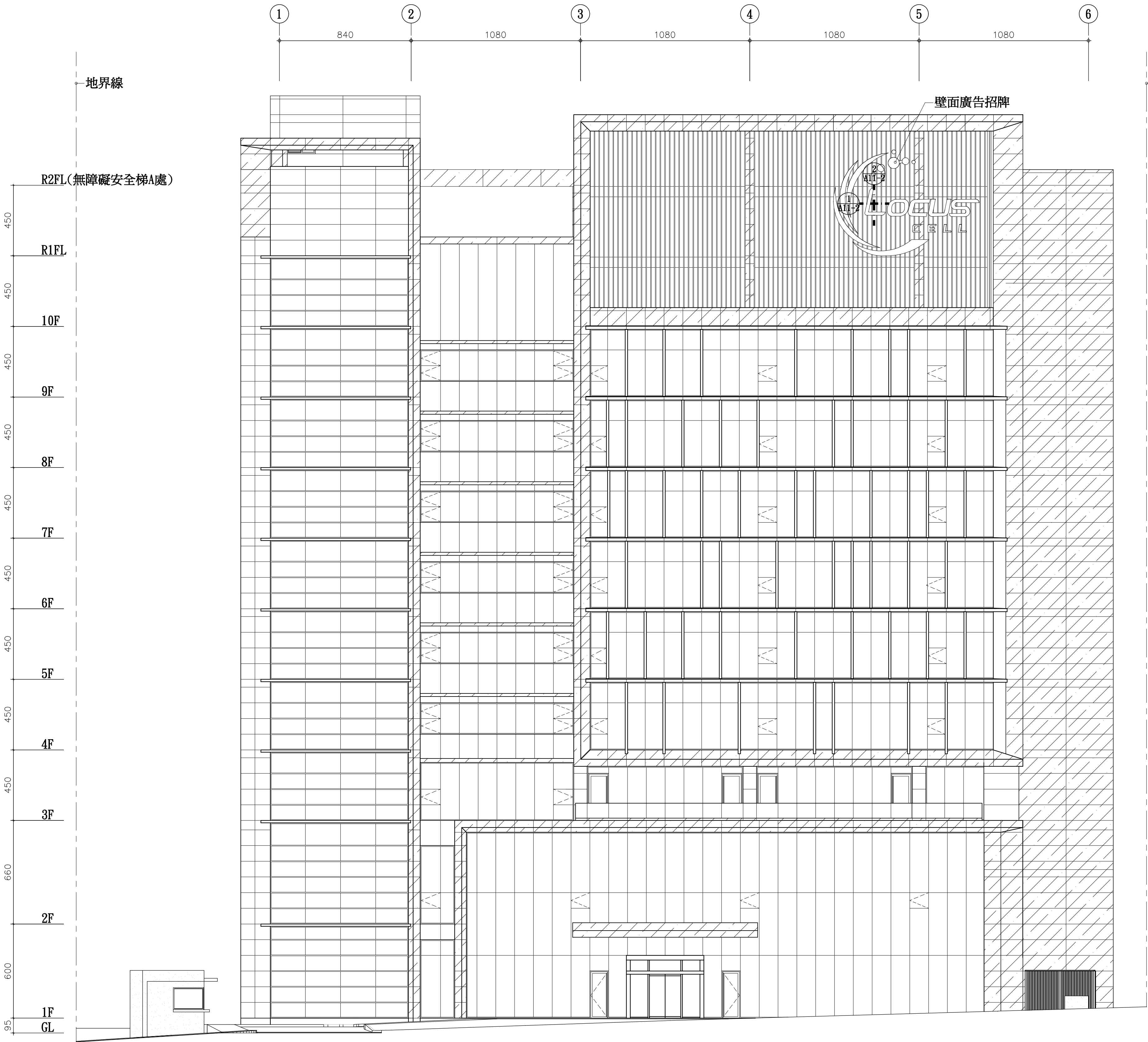
1 A11-1 西北向立面圖 A1=S:1/150 A3=S:1/300
