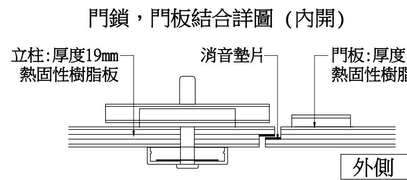
門鎖, 門板結合詳圖 (外開)
