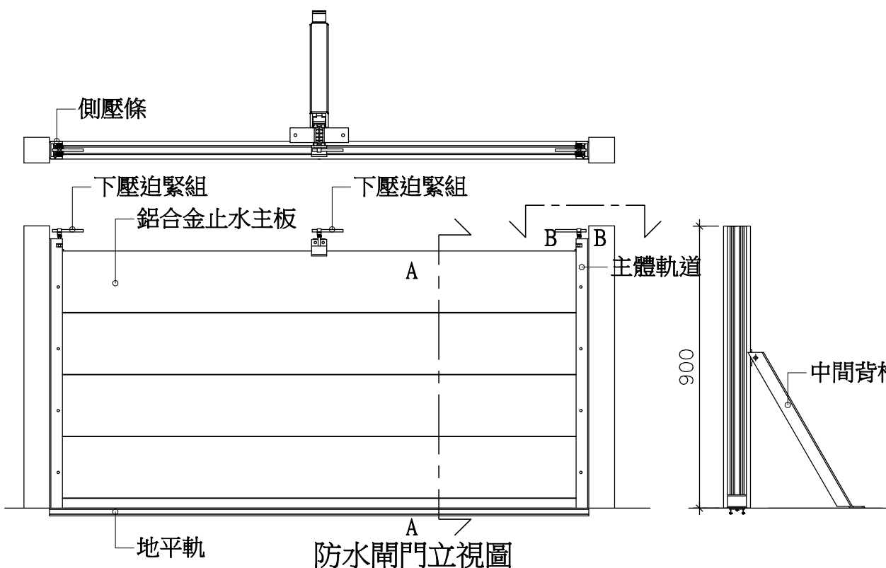
防水閘門立視圖
