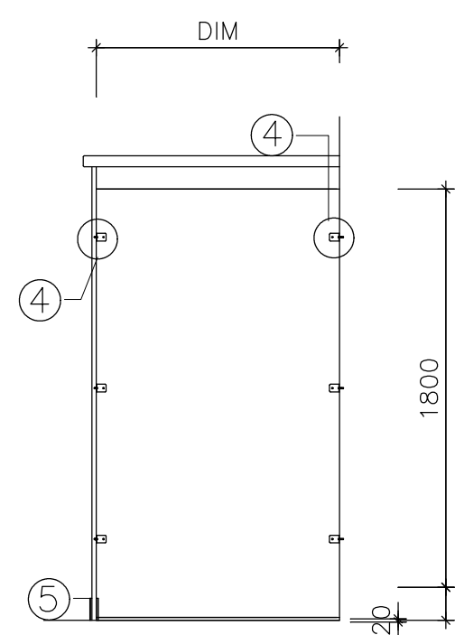
TYPE A內隔間板側立面圖
