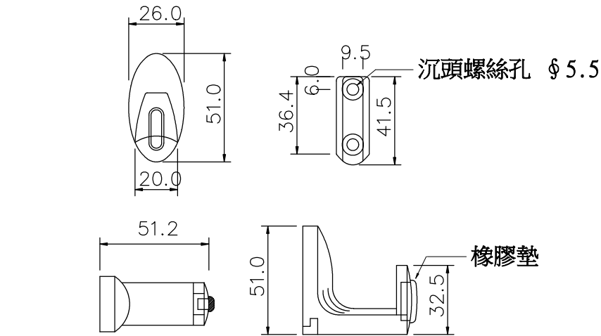
掛衣鉤 (鋅合金鍍鉻) 詳圖
