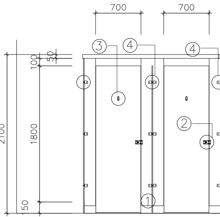
TYPE A背立面圖
