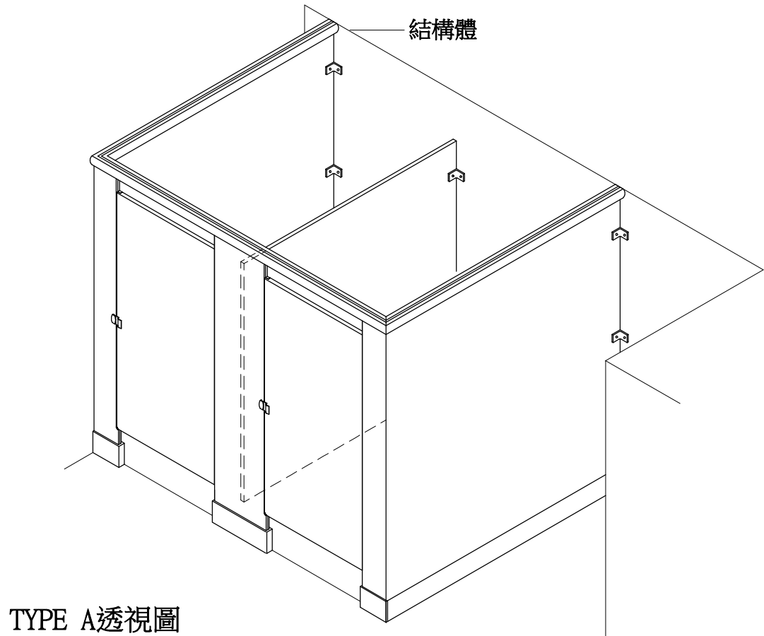
TYPE A透視圖
