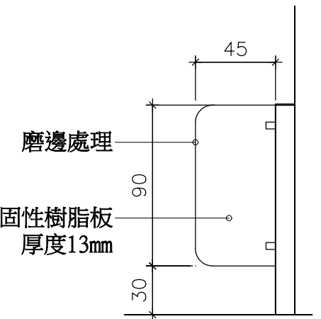
小便斗側立面圖
