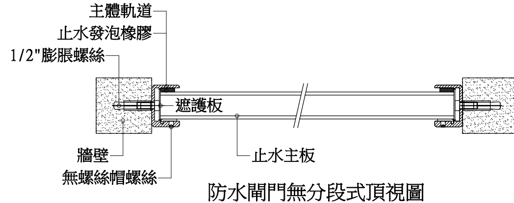
防水閘門無分段式頂視圖
