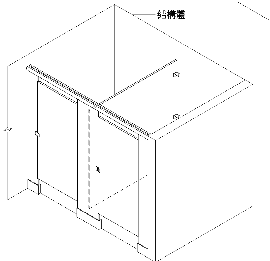
TYPE B透視圖
