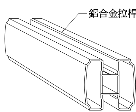
拉桿詳圖
