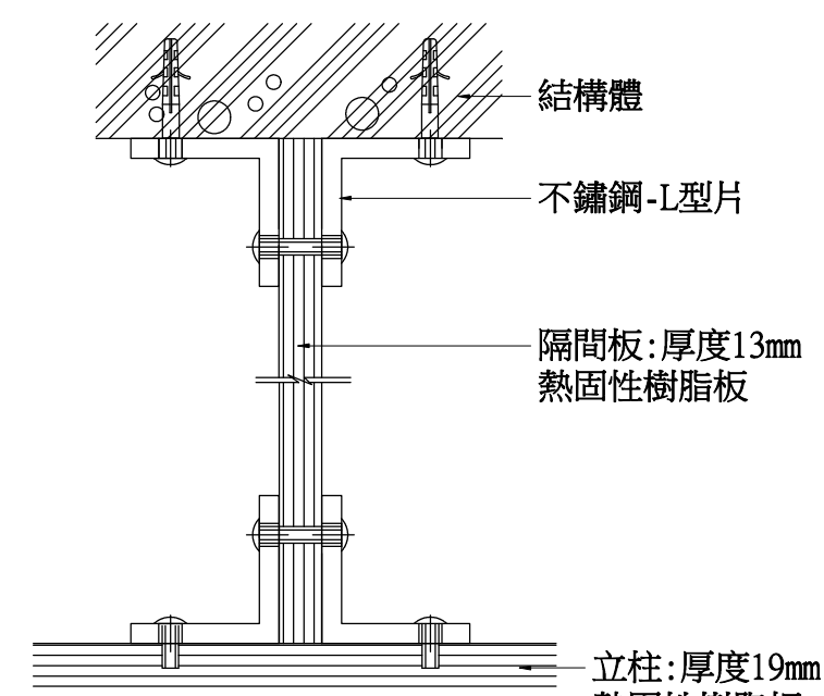
隔間板與立柱, 牆面結合詳圖
