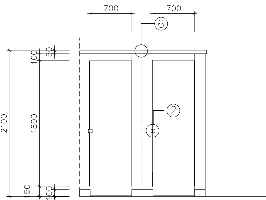
TYPE A正立面圖
