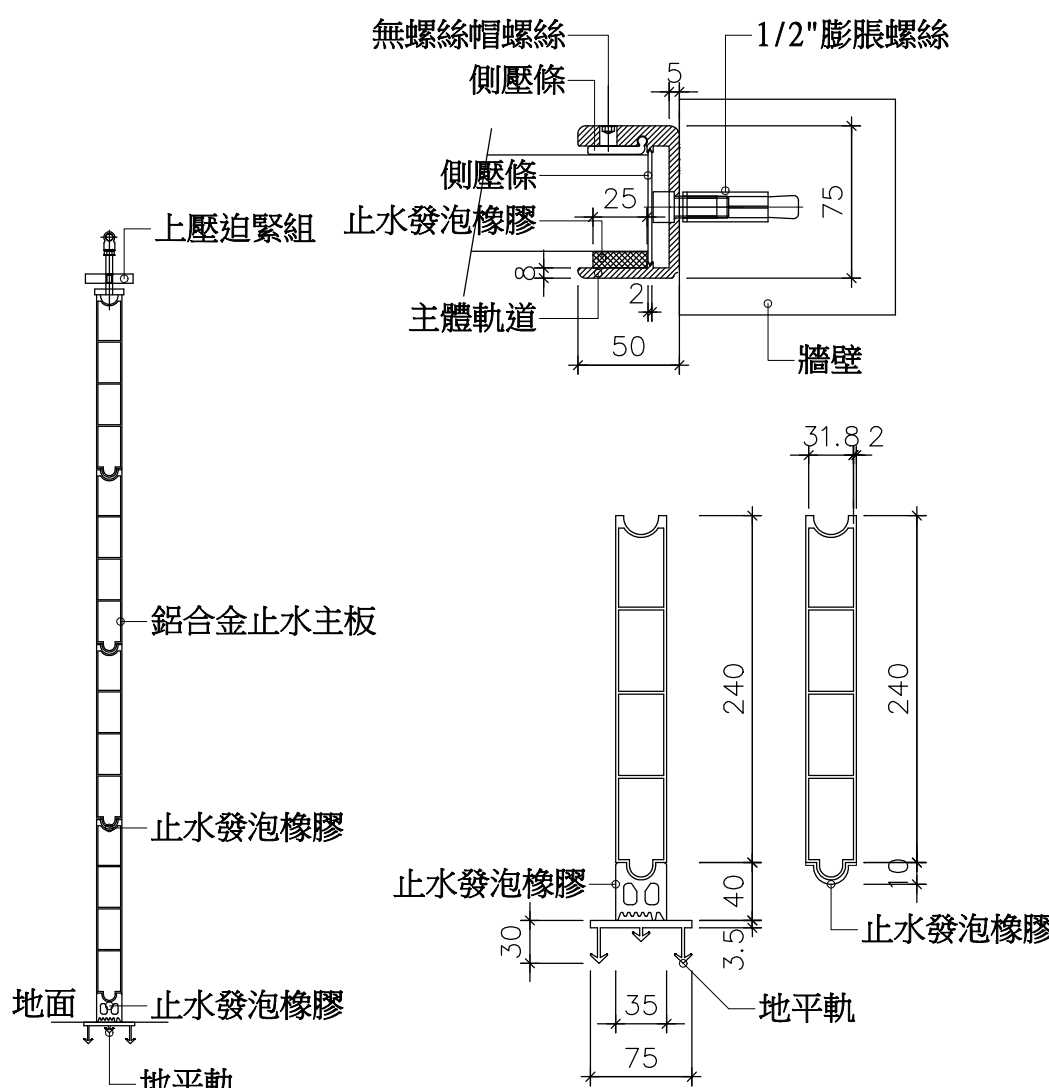
A-A VIEW
