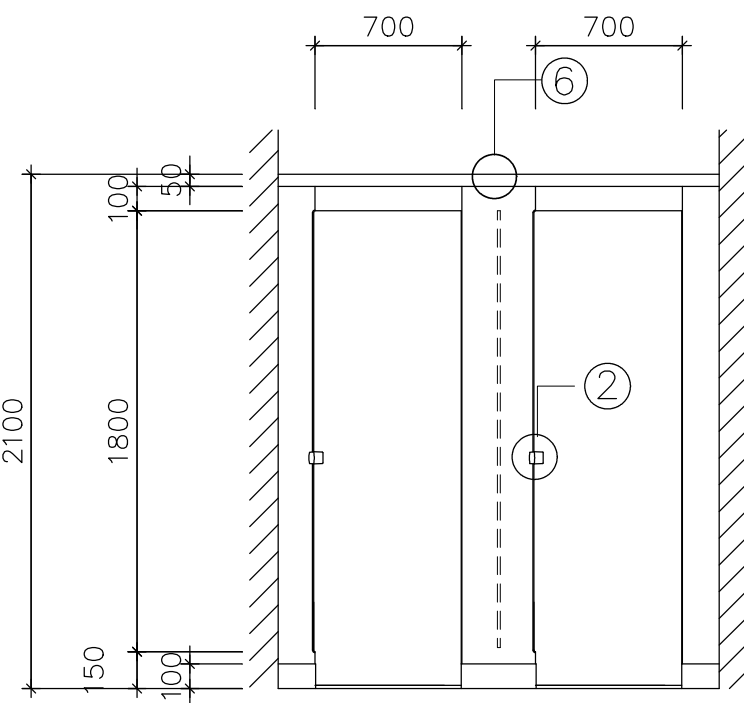
TYPE B正立面圖
