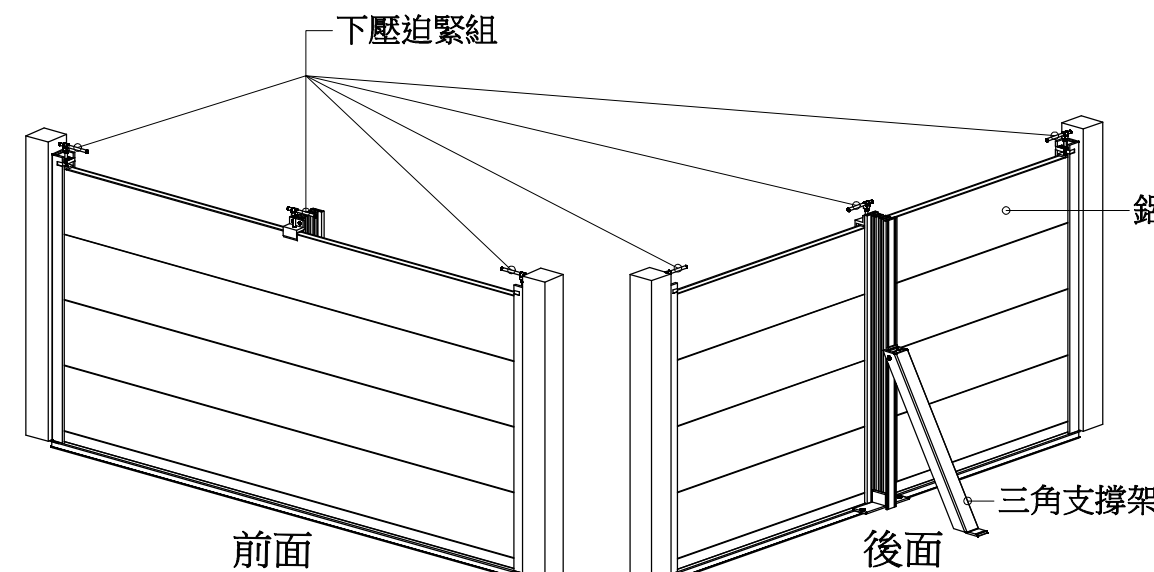
防水閘門無分段式立視圖
