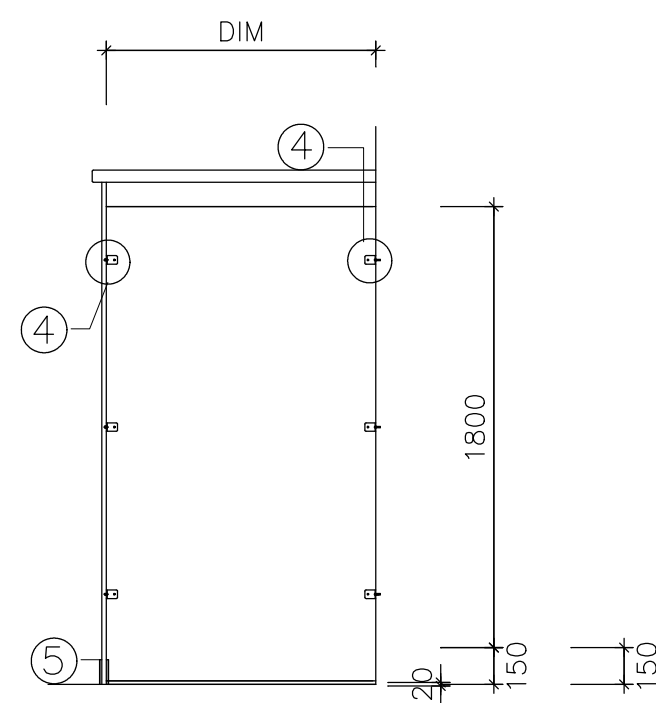
TYPE B內隔間板側立面圖
