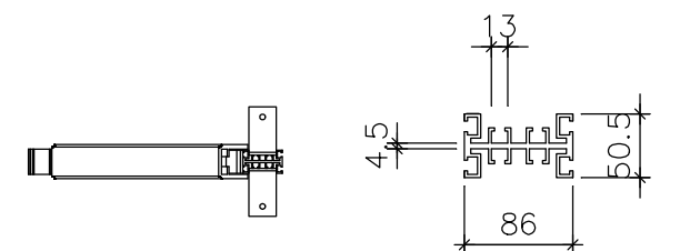
工字鐵尺寸, 高度視擋水主板片數而定
