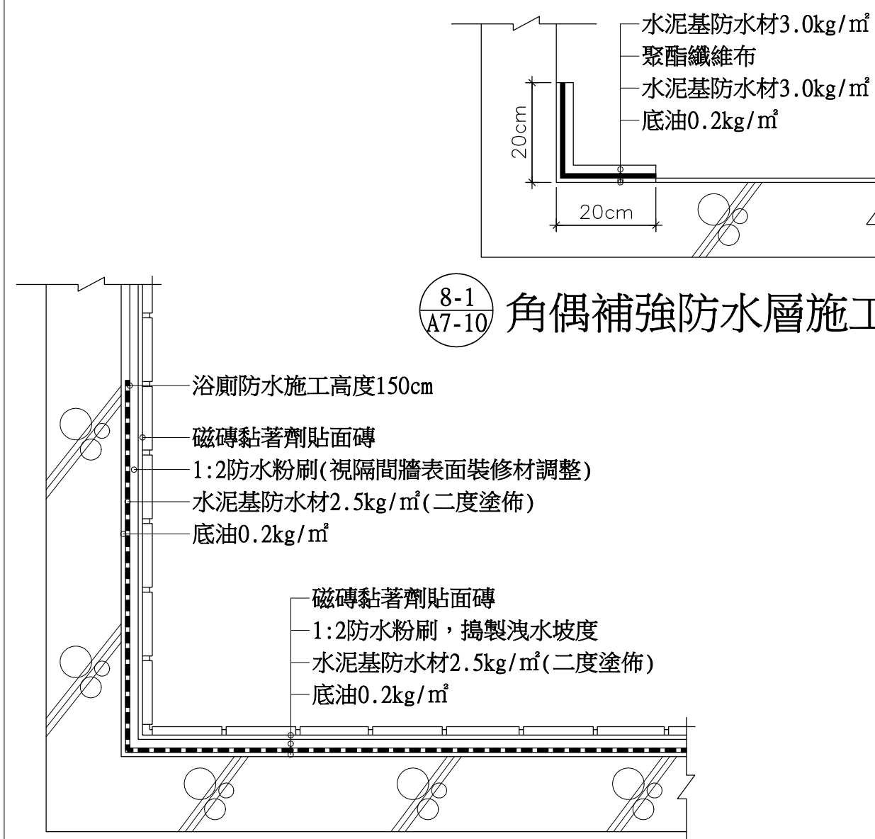
8 A7-1 浴廁地坪及牆面(RC牆)防水層施工詳圖
