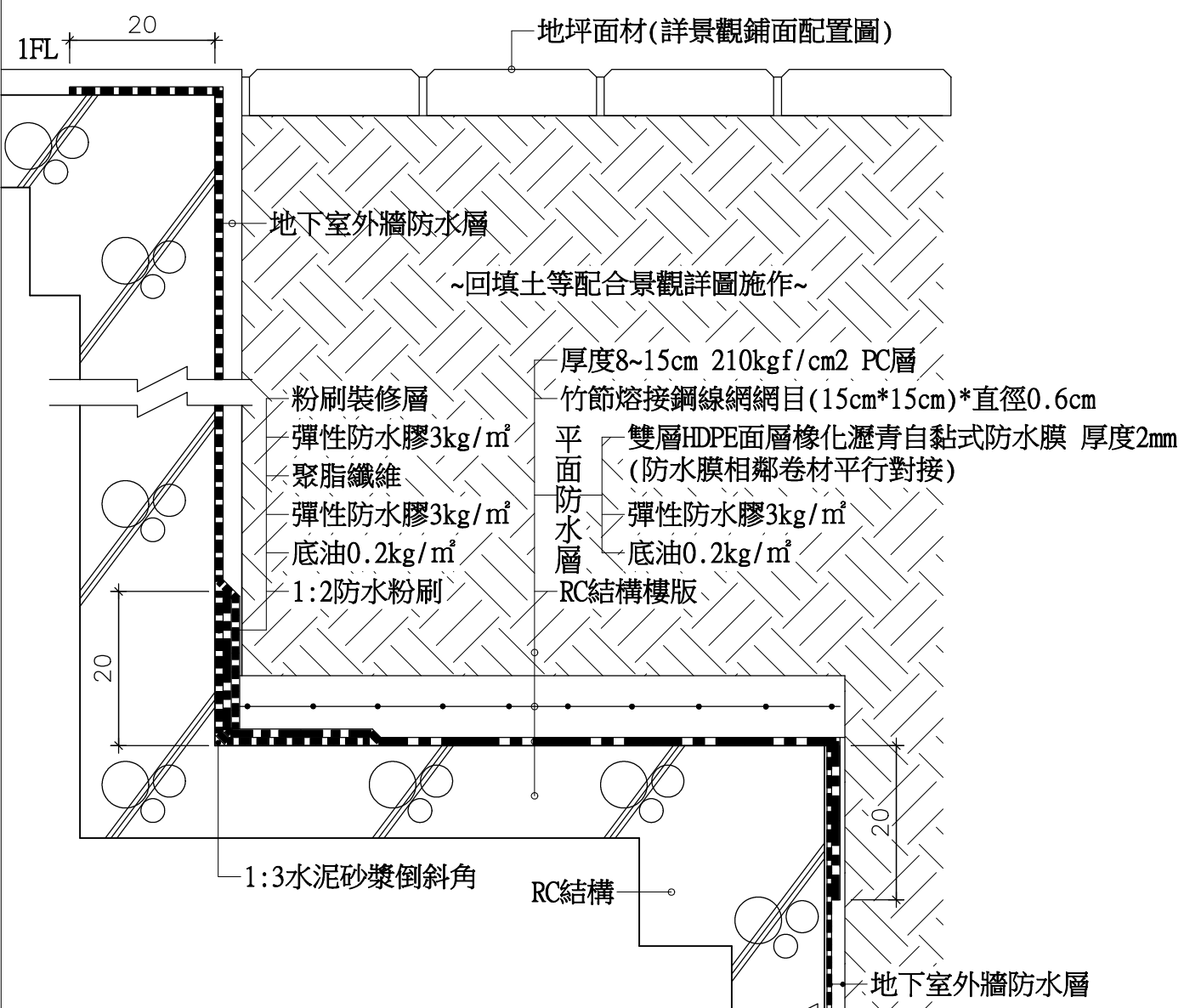
3 A7-1 地下室頂版防水層施工詳圖
