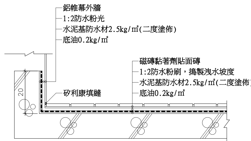
9 A7-1 陽台及裝卸平台地坪及牆面防水層施工詳圖
