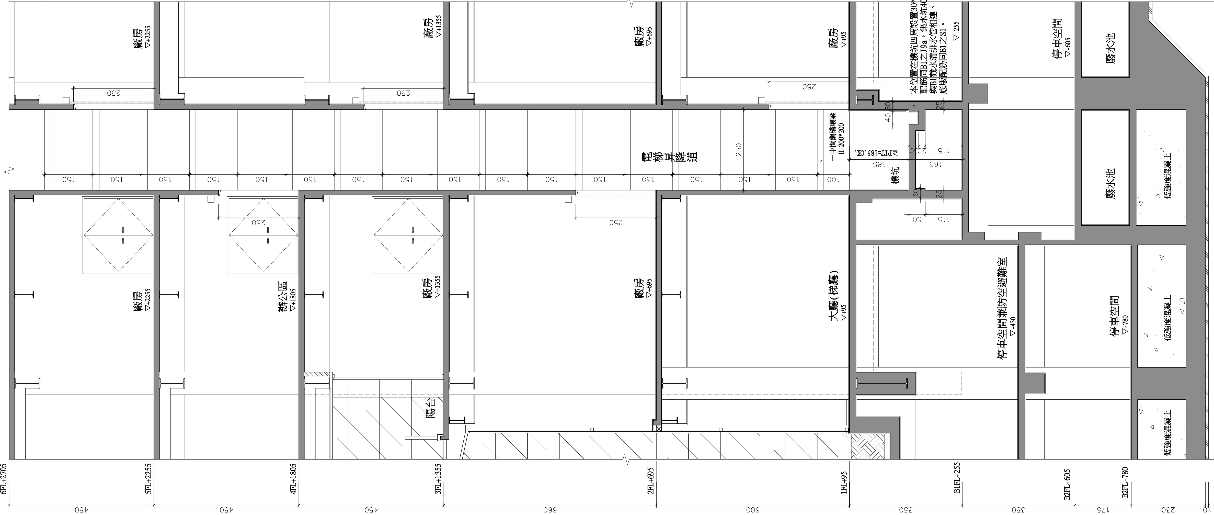
1 NO.5客貨梯昇降道剖面圖(一) A1=S:1/60 A3=S:1/120
