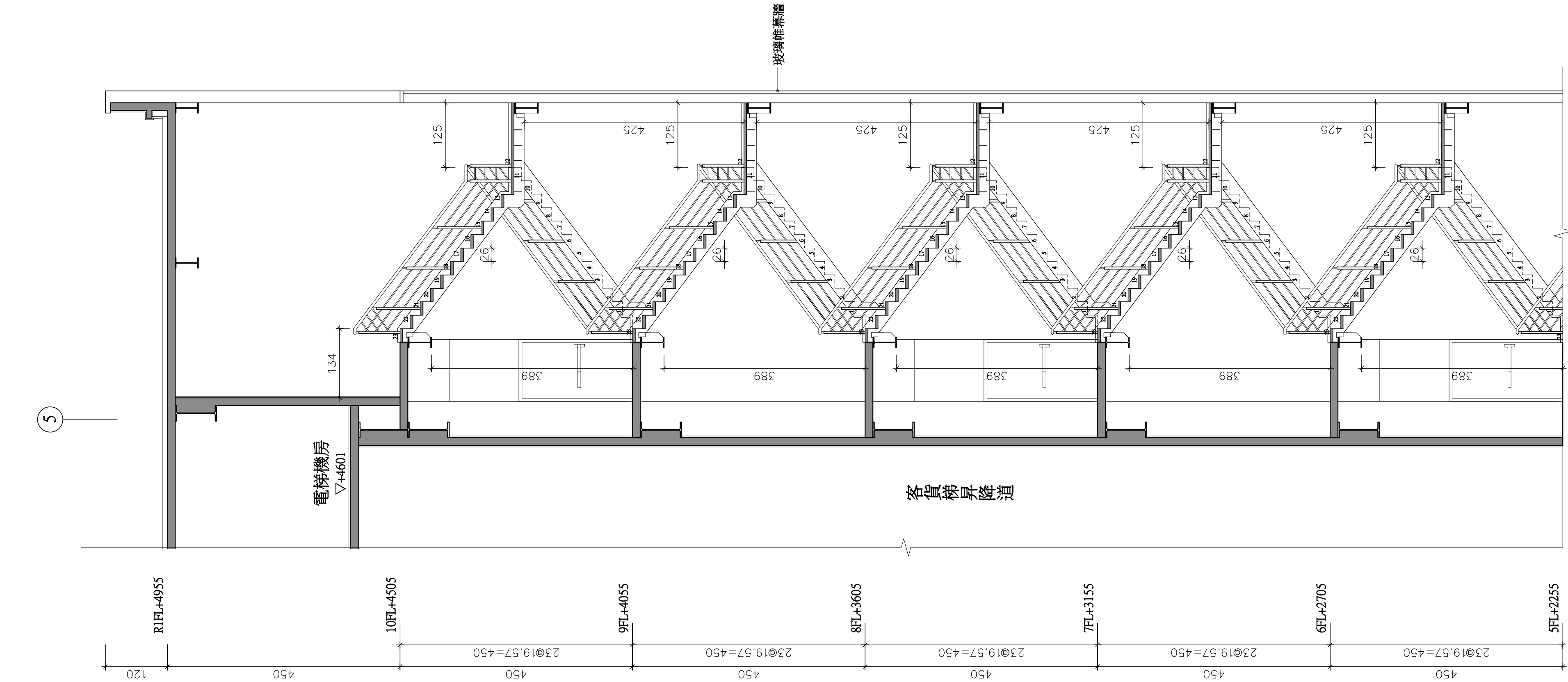
安全梯C剖面圖(二) A1=S:1/60 A3=S:1/120
