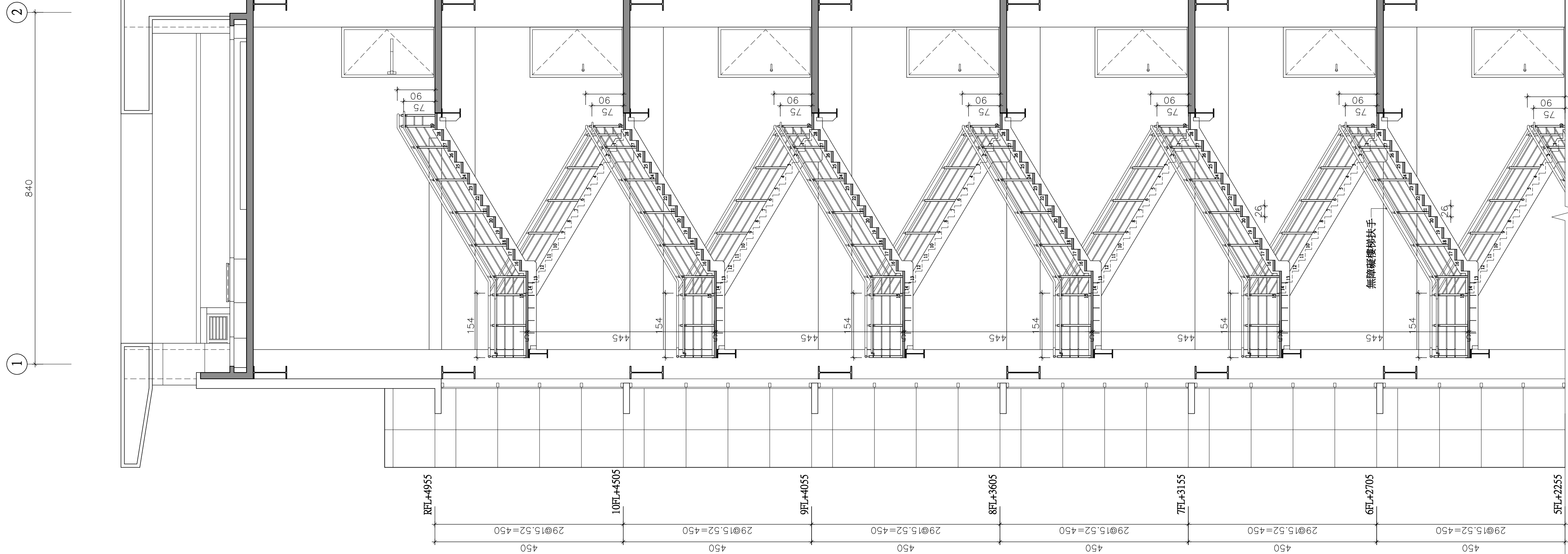
2 A4-3 無障礙安全梯A剖面圖(二) A1=S:1/60 A3=S:1/120
