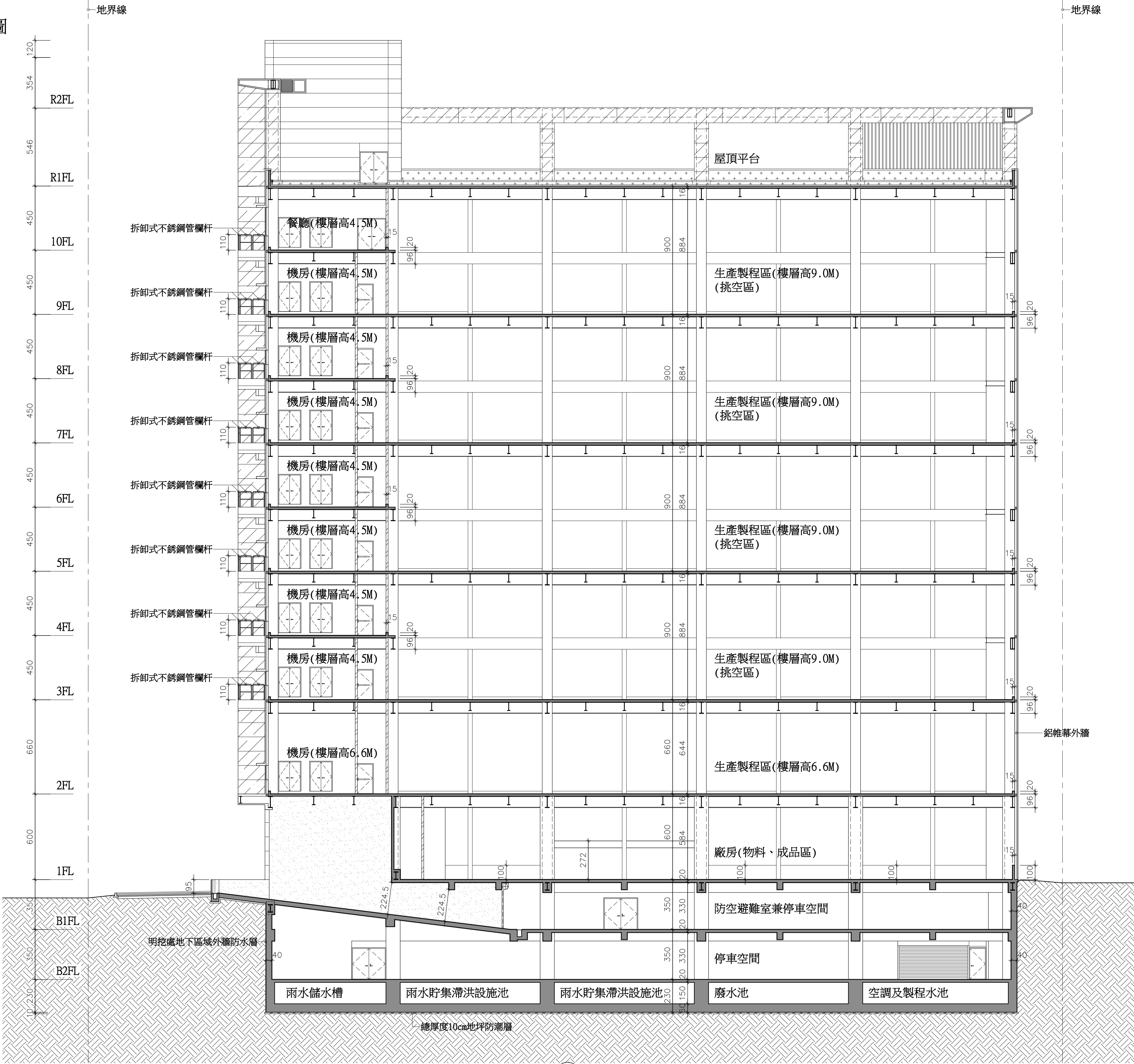
南北向剖面圖 A1=S:1/150 A3=S:1/300
