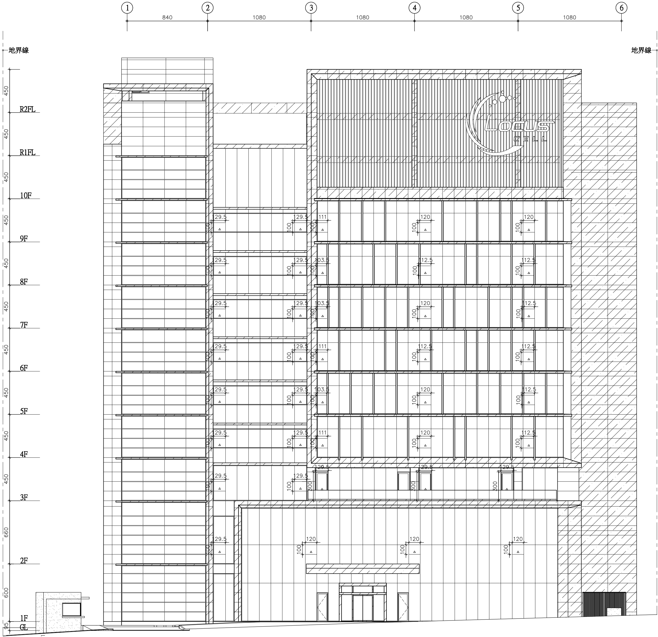
1 A3-5 西北向立面圖 A1=S:1/200 A3=S:1/400
