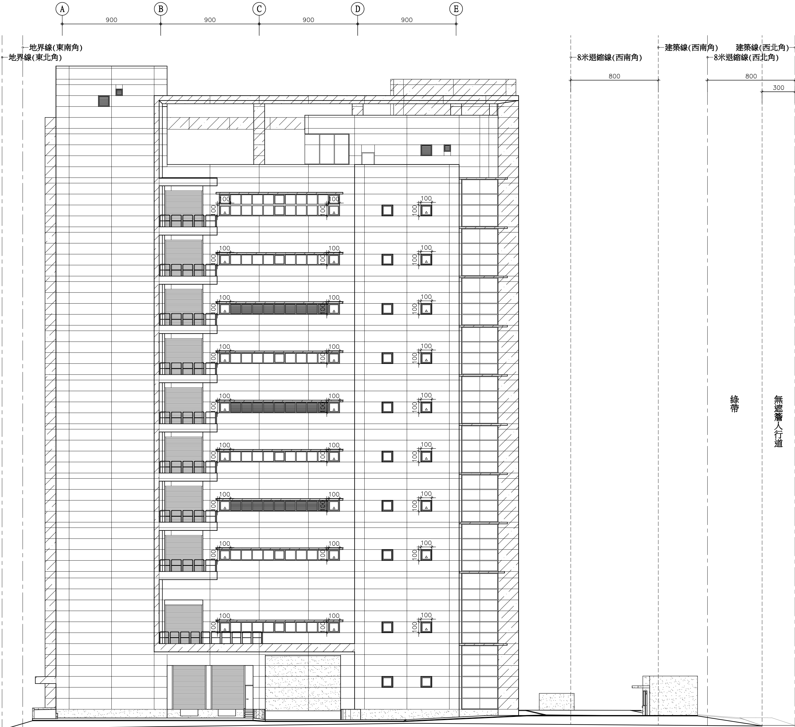
2 A3-5 東北向立面圖 A1=S:1/200 A3=S:1/400
