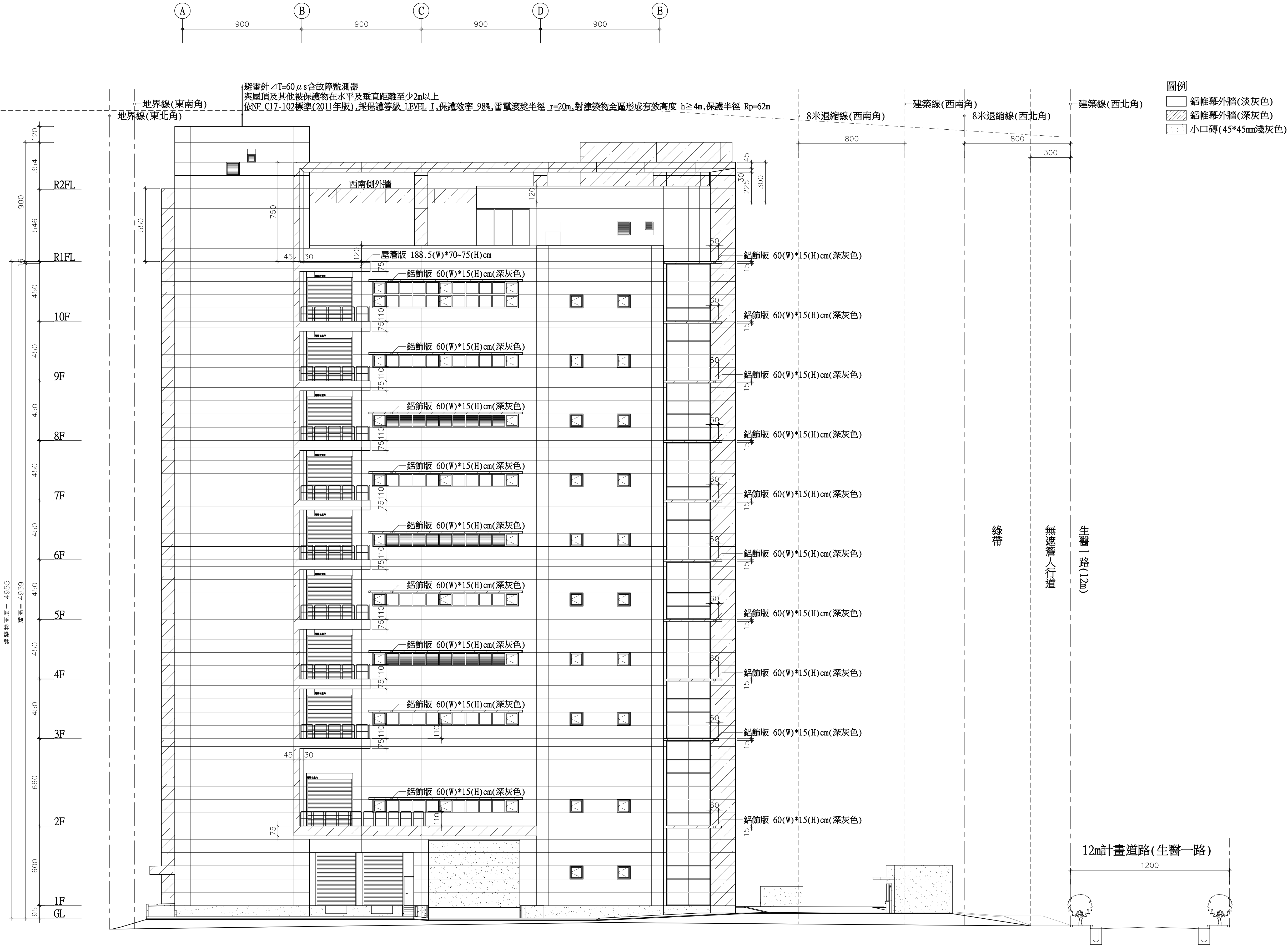
1 A3-3 東北向立面圖 A1=S:1/150 A3=S:1/300
