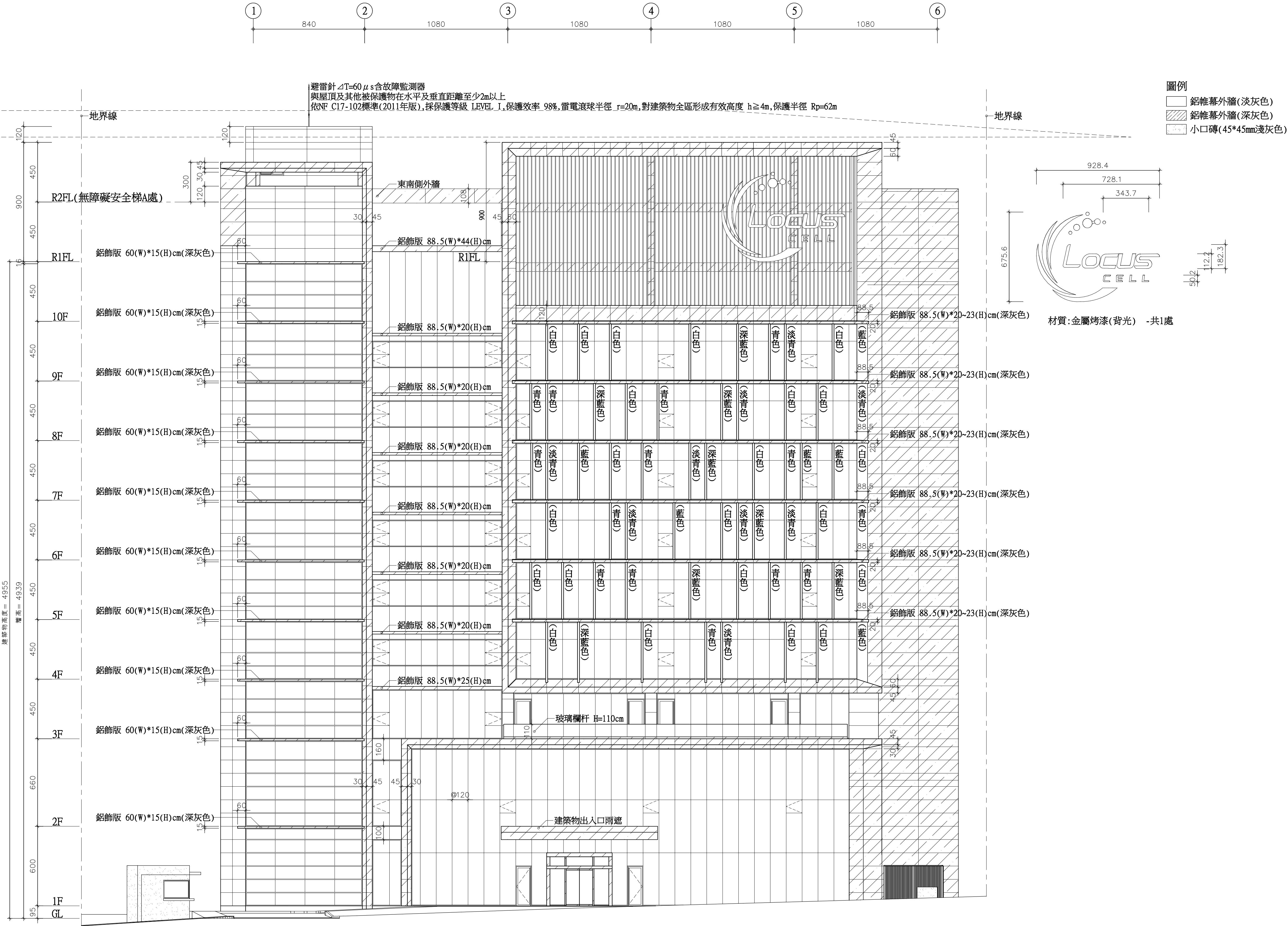
1 A3-1 西北向立面圖 A1=S:1/150 A3=S:1/300
