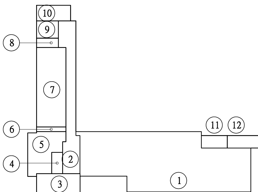
四層防火區劃檢討圖 檢討計算式詳見A1-10
