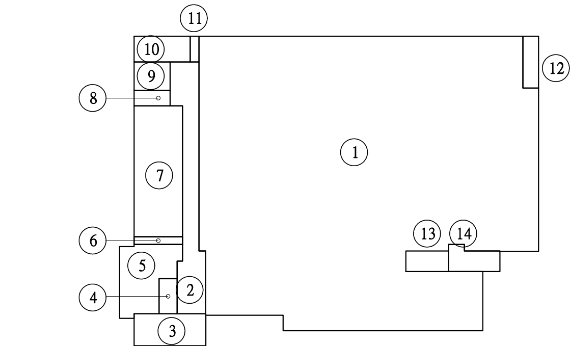
三層防火區劃檢討圖 檢討計算式詳見A1-10
