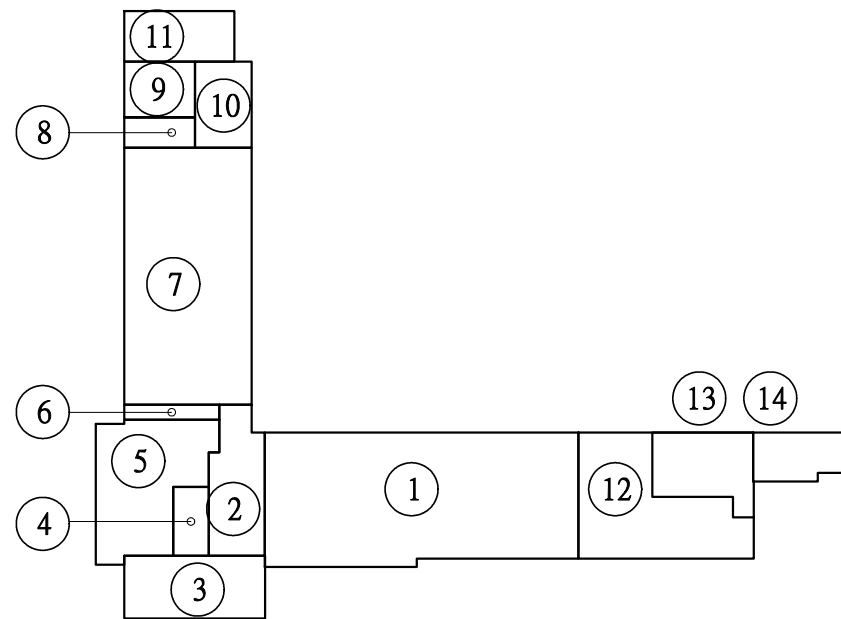
十層防火區劃檢討圖 檢討計算式詳見A1-11
