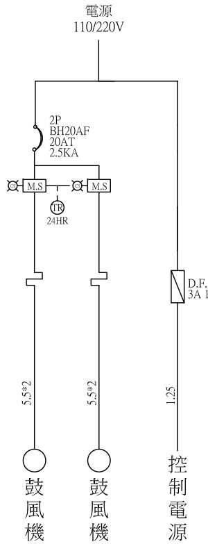
單線圖
