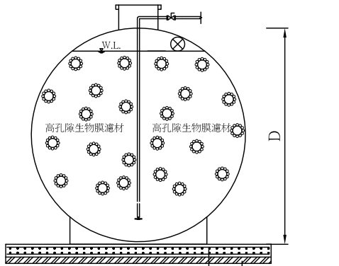
剖面圖
