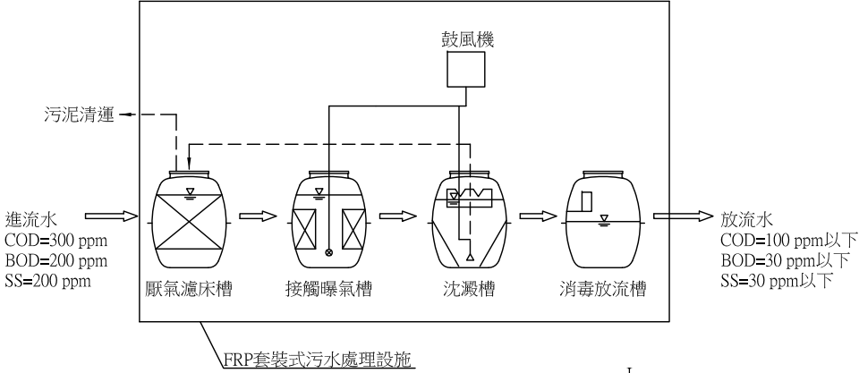
流程圖
