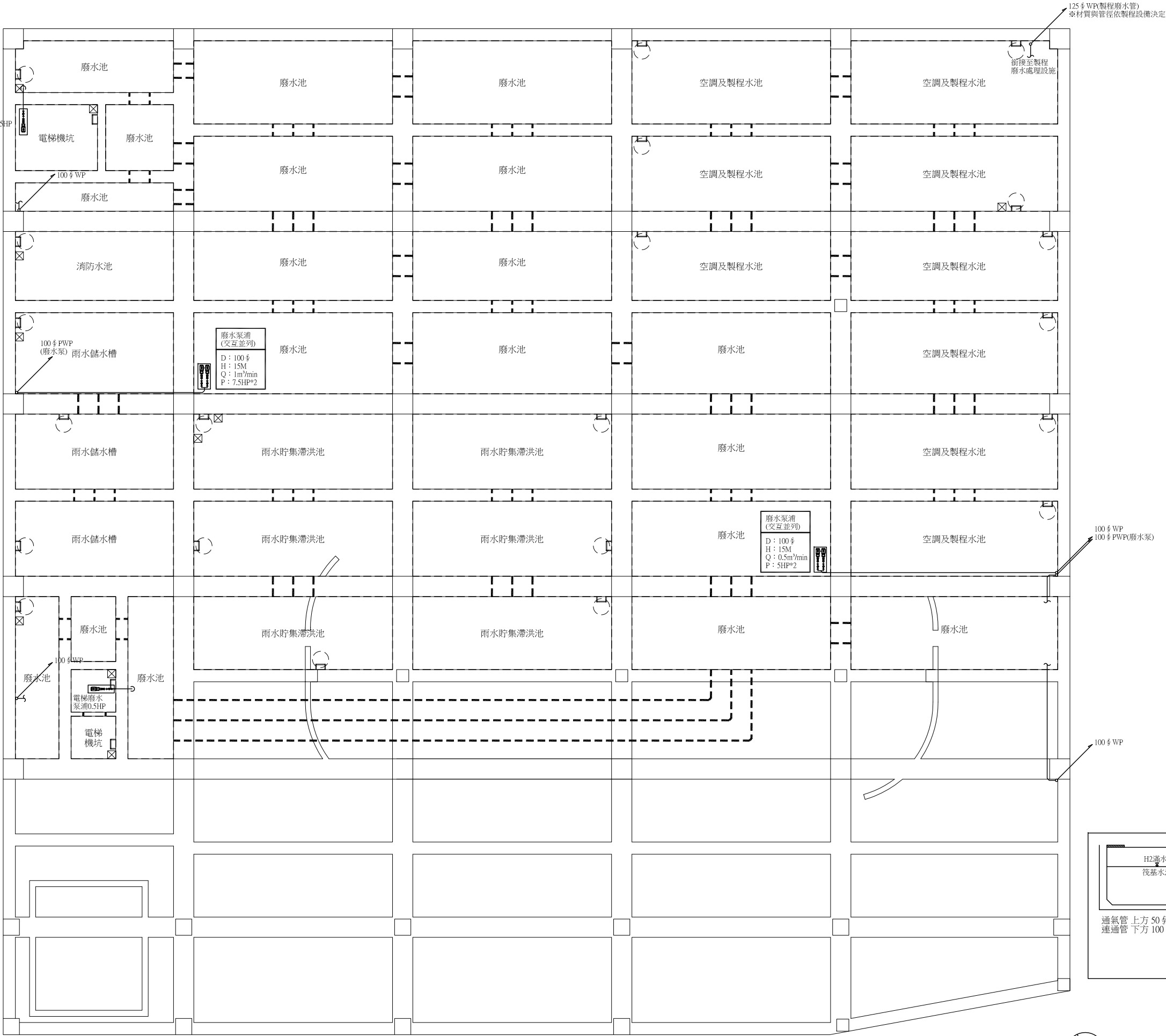
筏基層排水平面圖 A1=S:1/100
