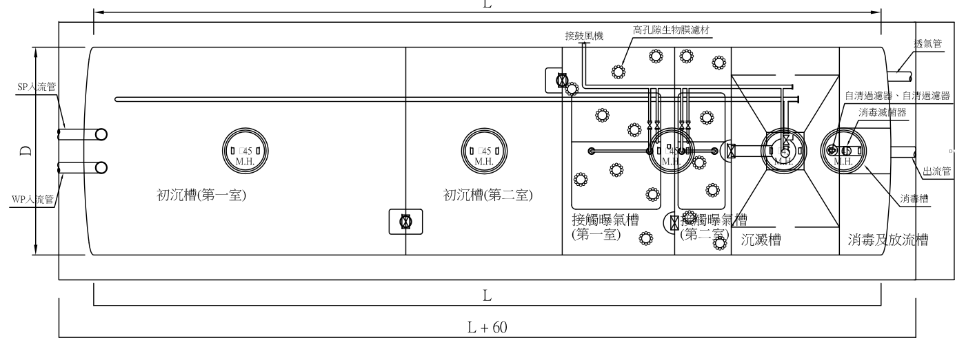
平面圖
