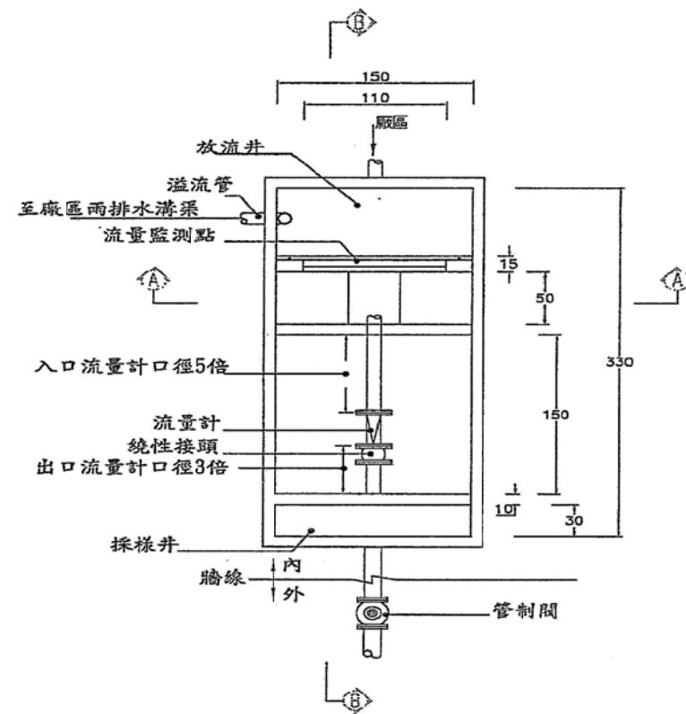
計量槽及採樣井平面圖
