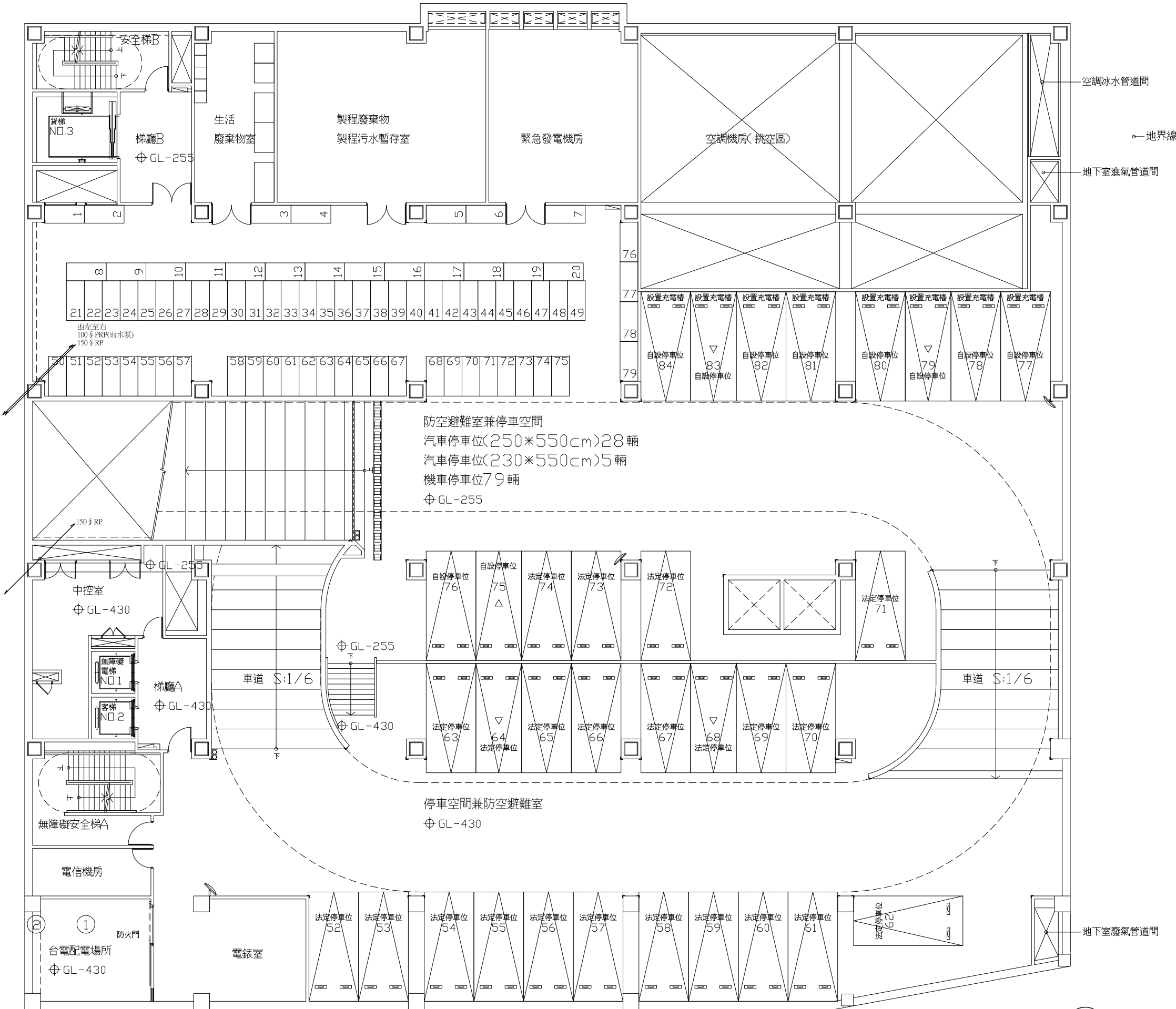
地下一層雨水平面圖 A1=S:1/100
