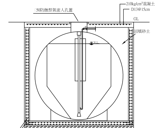
混凝土防護示意圖
