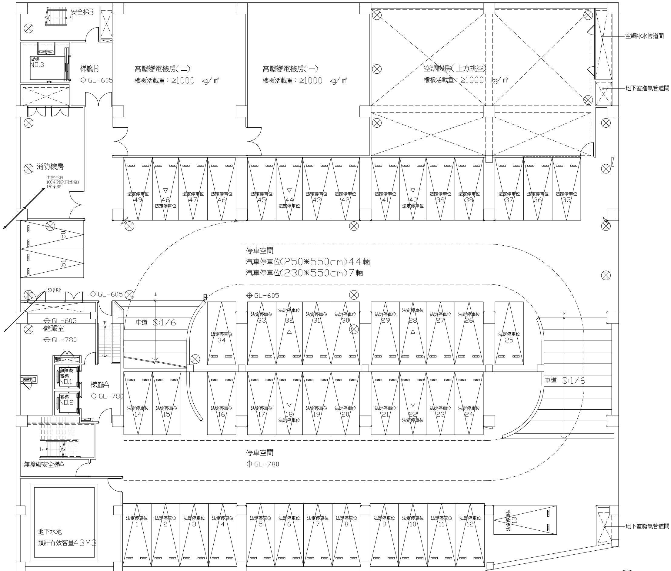
地下二層雨水平面圖 A1=S:1/100
