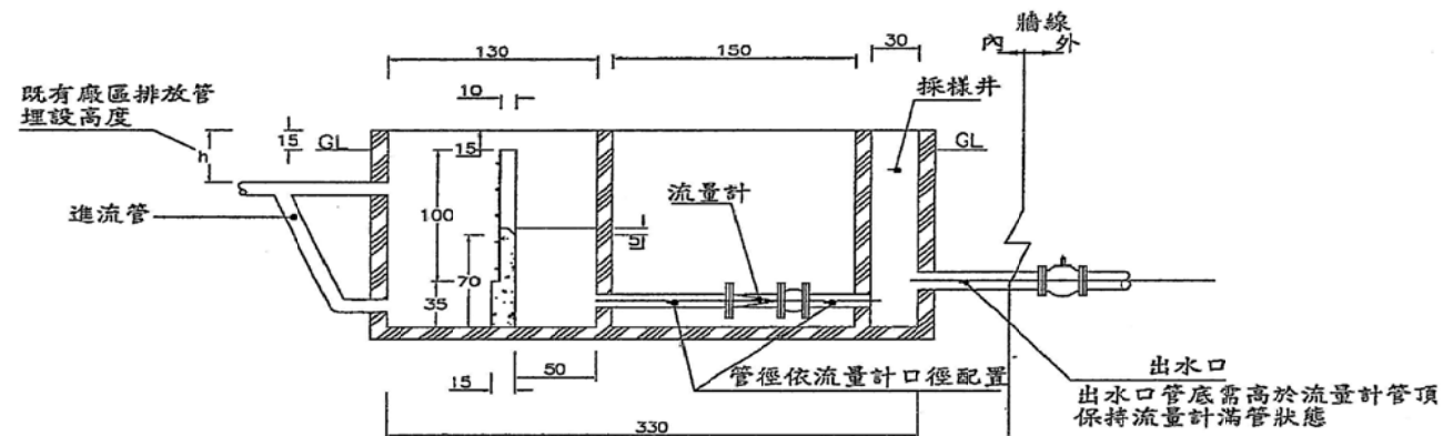
計量槽及採樣井B-B剖面圖
