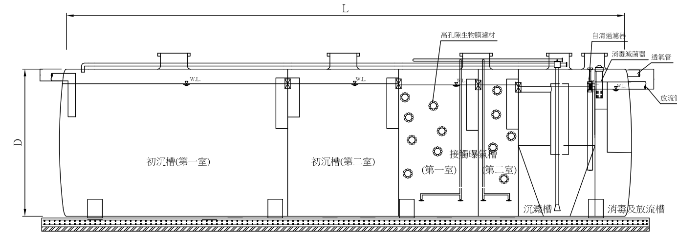
剖面圖
