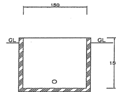
採樣井安裝圖
