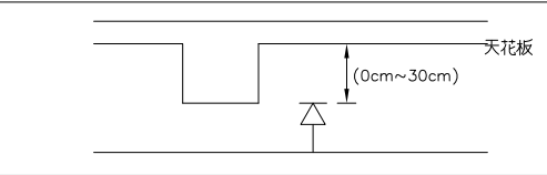
自動泡沫滅火設備一齊開放閥配置圖
