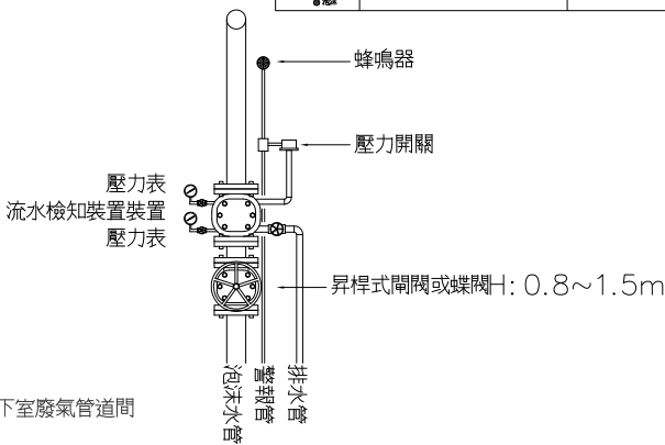
流水檢知裝置示意圖
