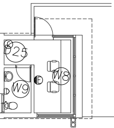
警衛室一層消防平面圖 S=1/200
