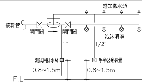
自動泡沫滅火設備一齊開放閥配置圖
