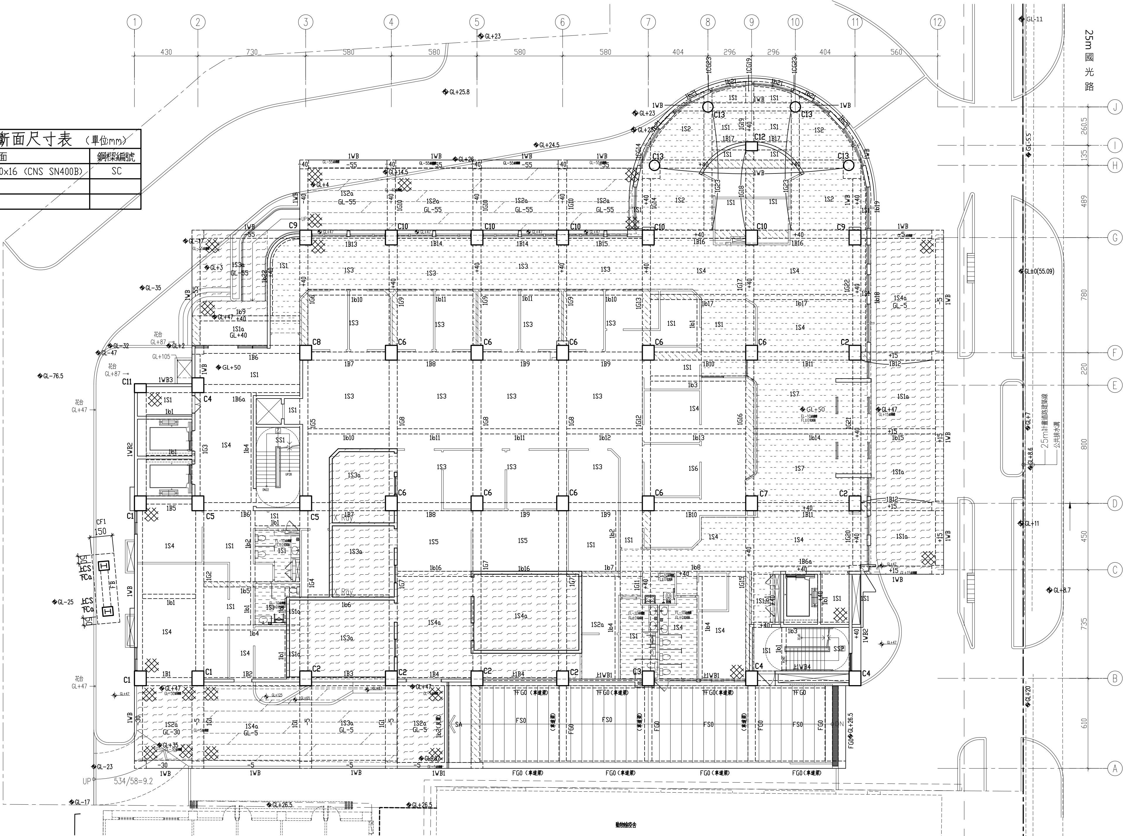
壹層結構平面圖
