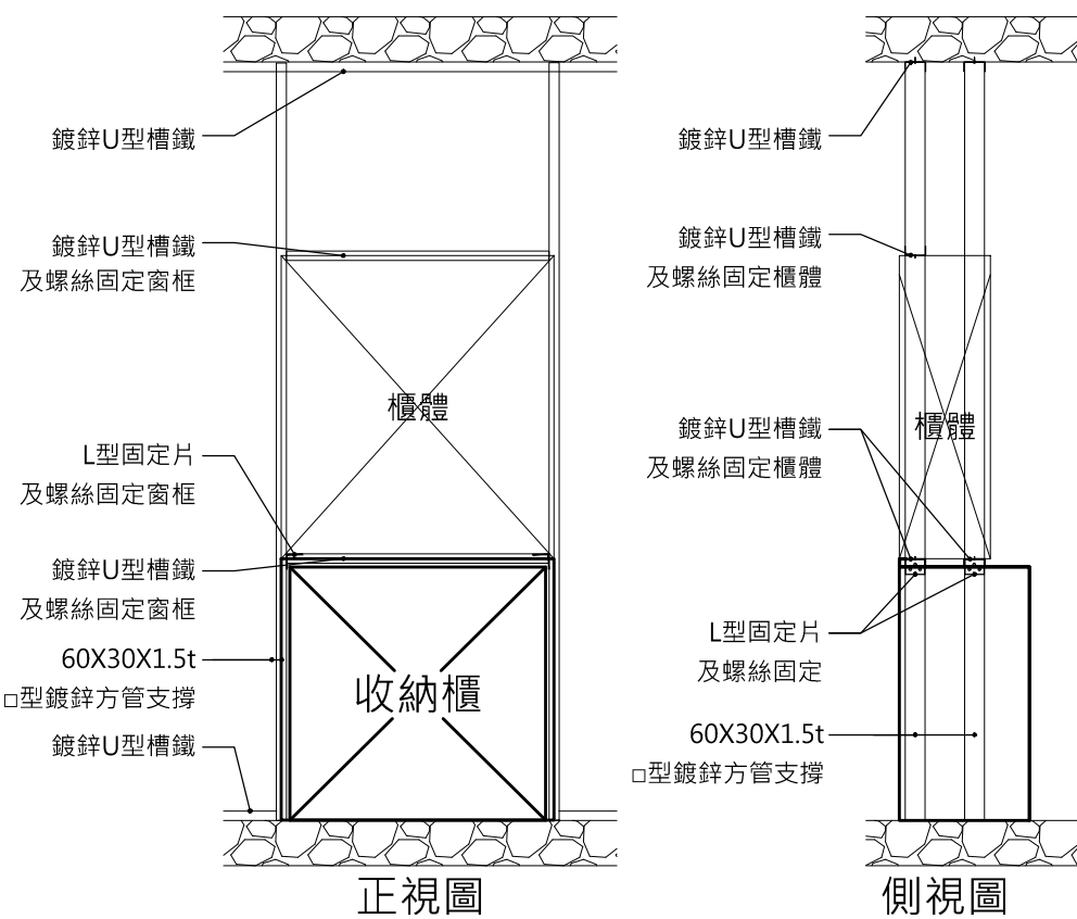
櫃體支撐補強(下方相連櫃體)施工詳圖
