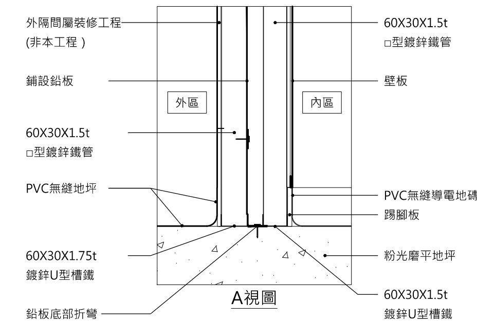
壁面、地坪縱剖面施工詳圖
