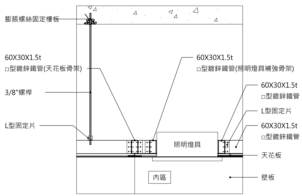
天花板.照明燈具縱剖面施工詳圖
