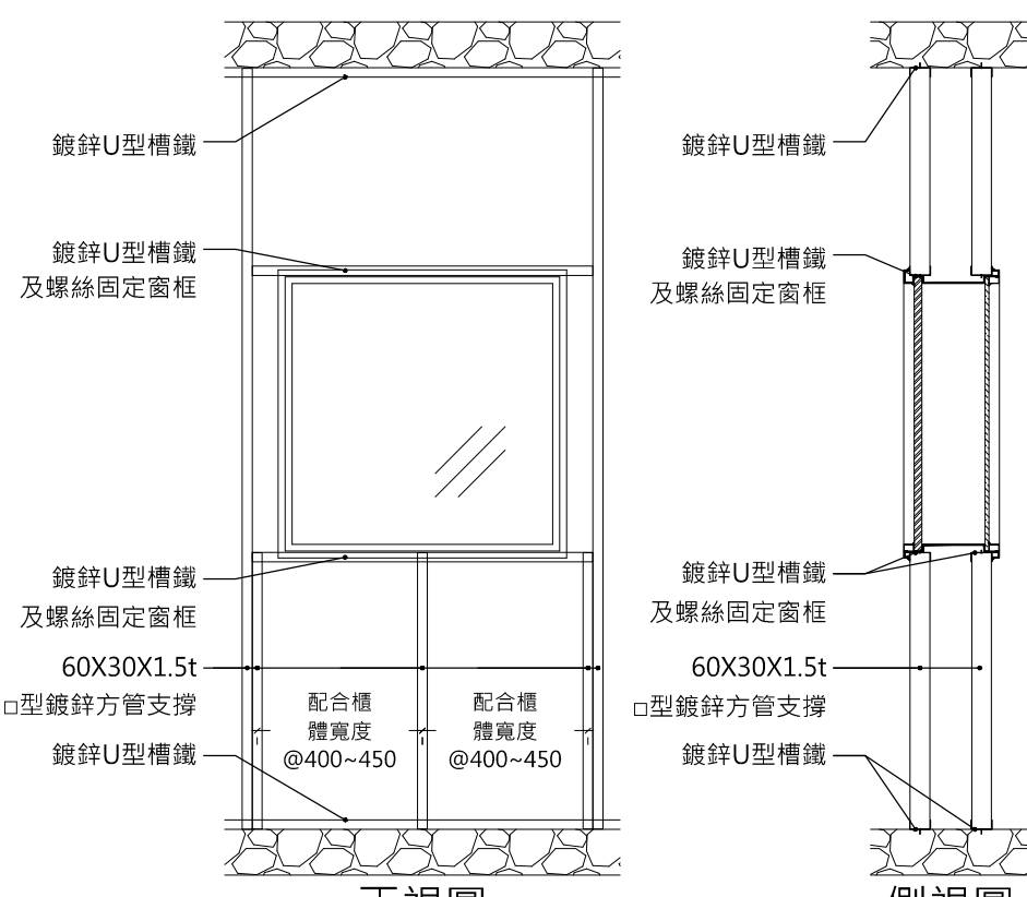
視窗支撐補強施工詳圖
