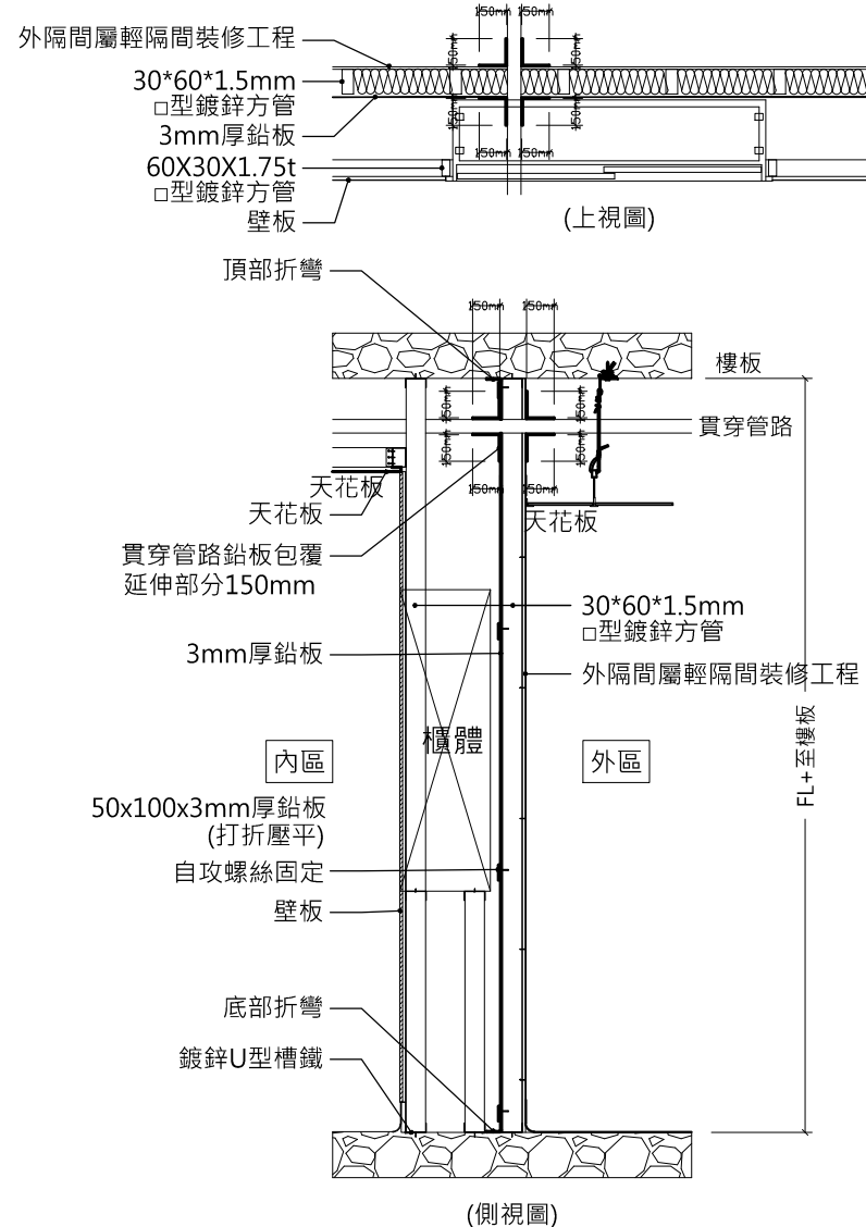
鉛板壁面剖面施工詳圖
