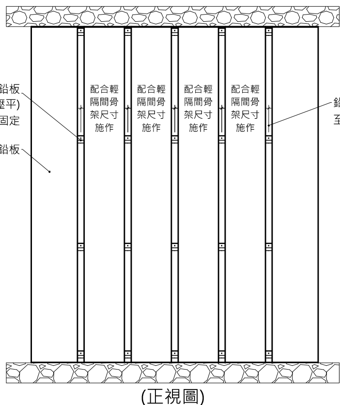
鉛板搭接重疊處壁面施工詳圖
