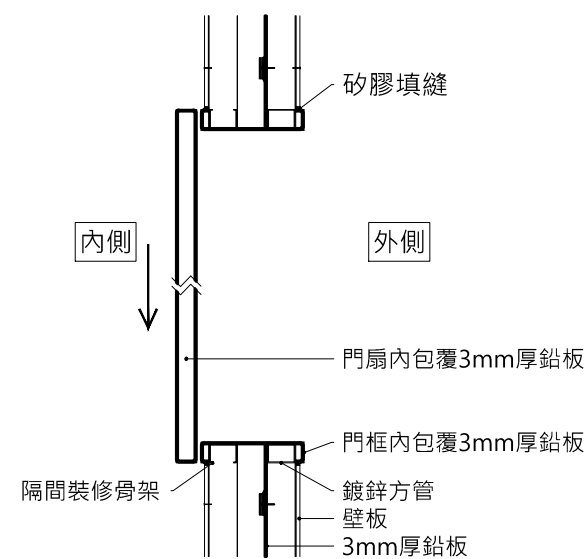
鉛板門剖面施工詳圖
