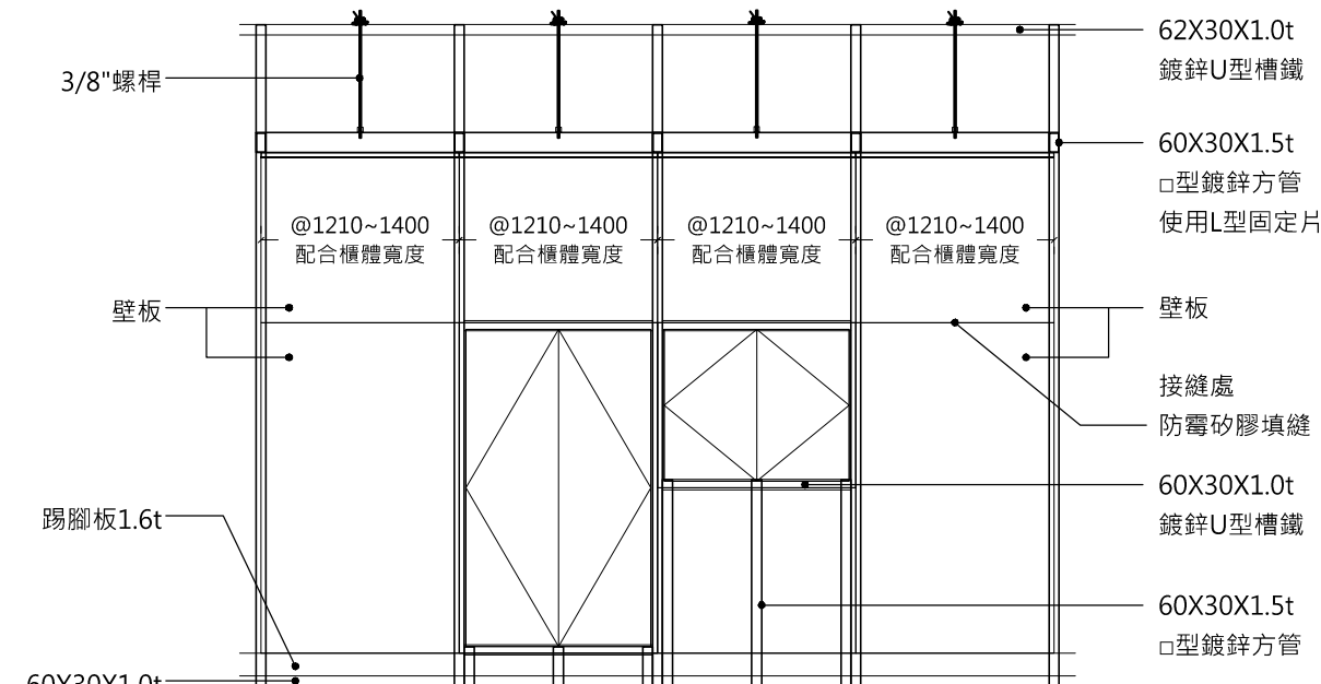
固定隔間立面施工詳圖
