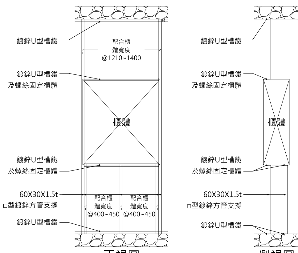
櫃體支撐補強施工詳圖
