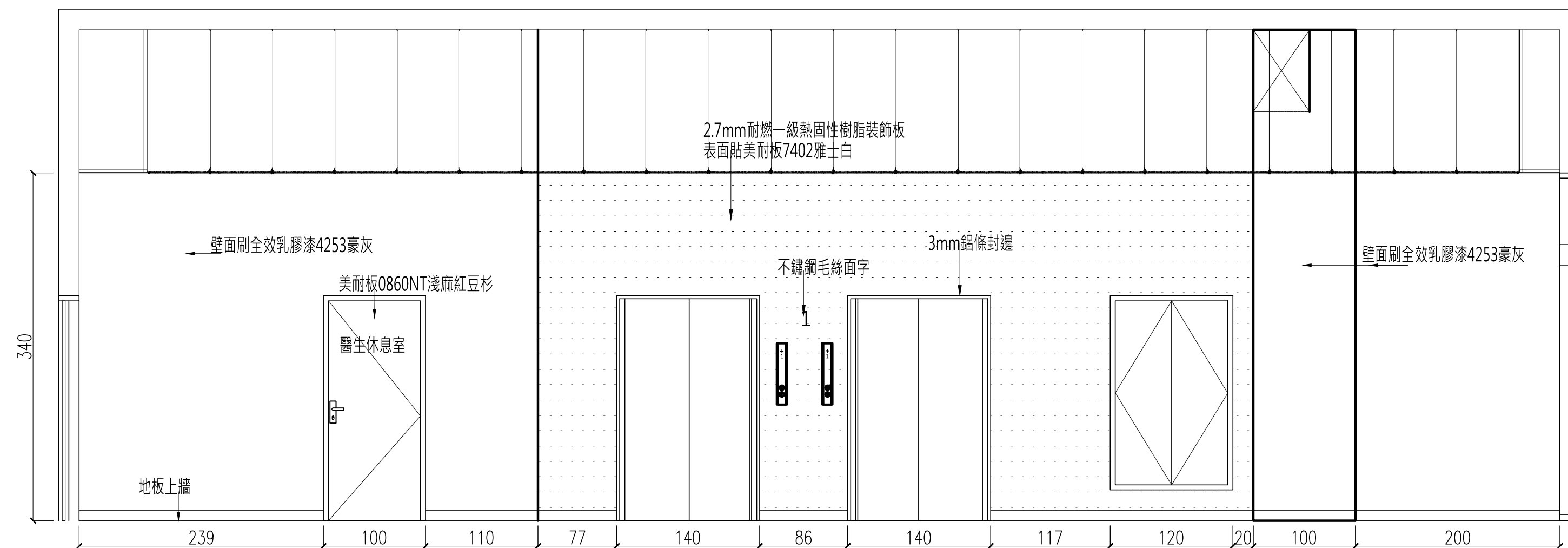
5 立面圖 S:1/40
