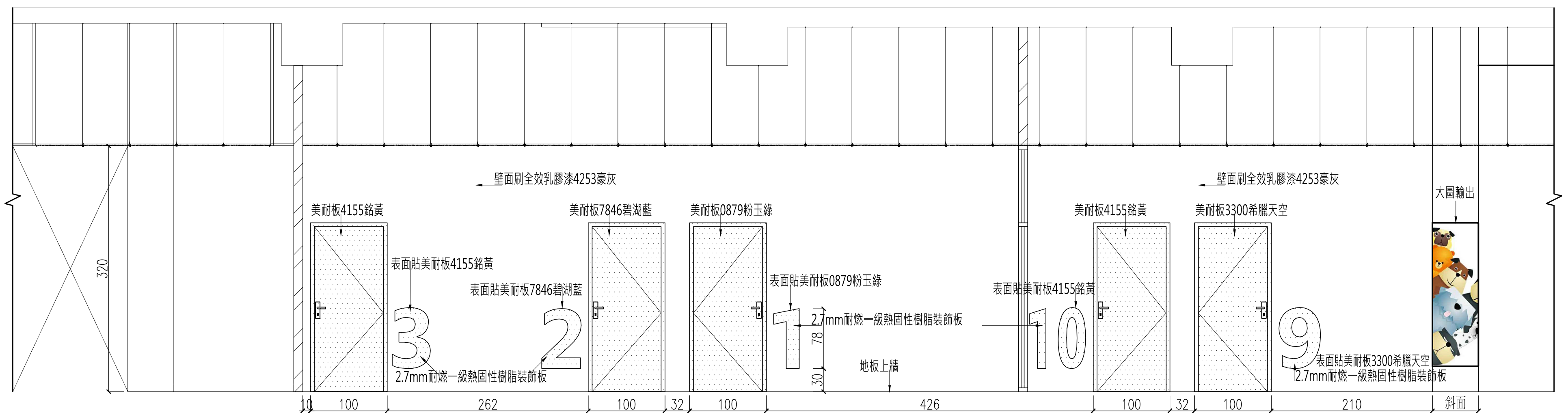
4 立面圖 S:1/40
