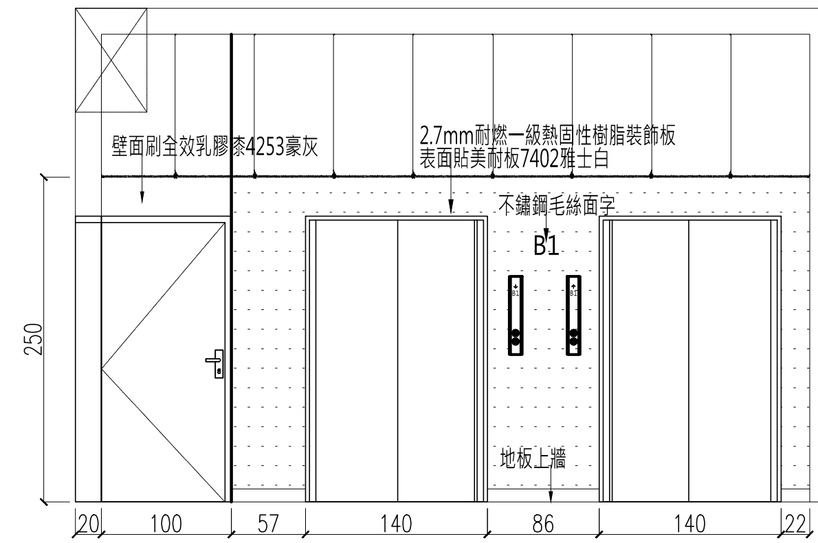
4a 立面圖 S:1/40
