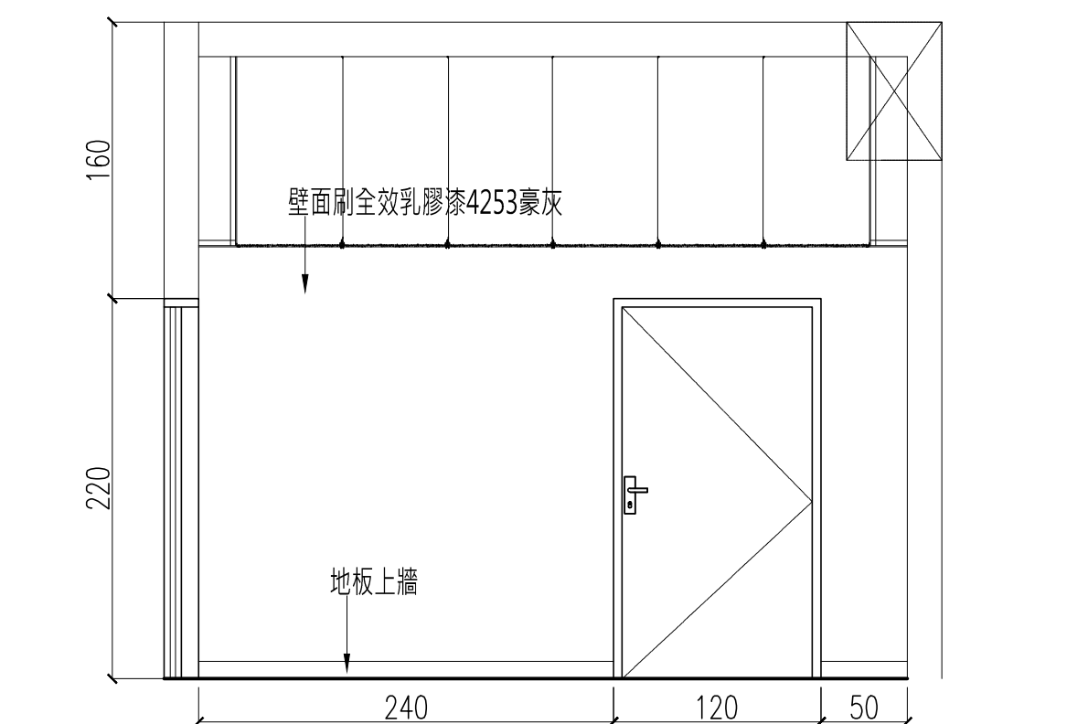
1d 立面圖 S:1/40
