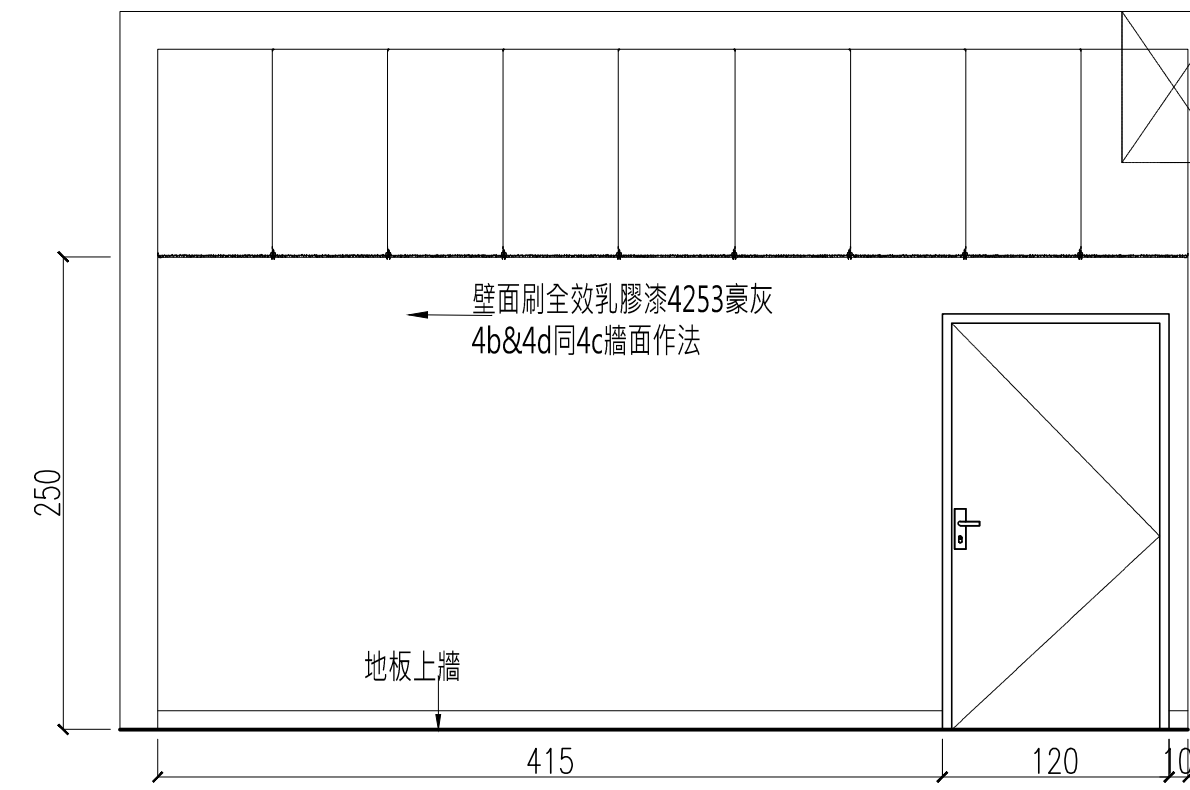
4c 立面圖 S:1/40
