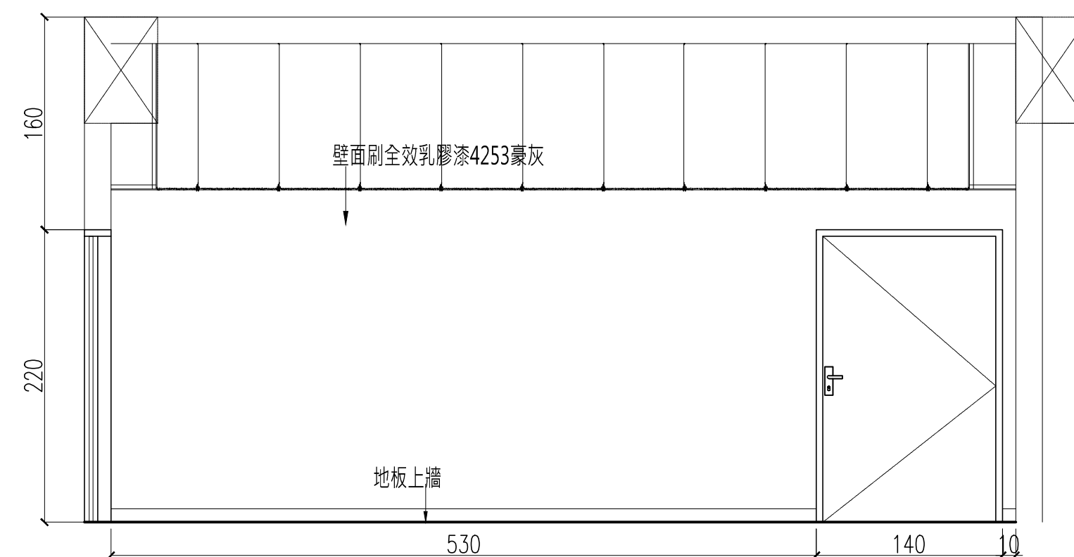
1c 立面圖 S:1/40
