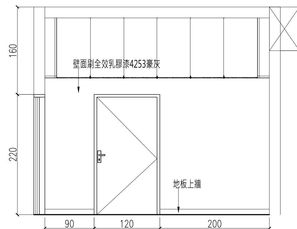
1b 立面圖 S:1/40
