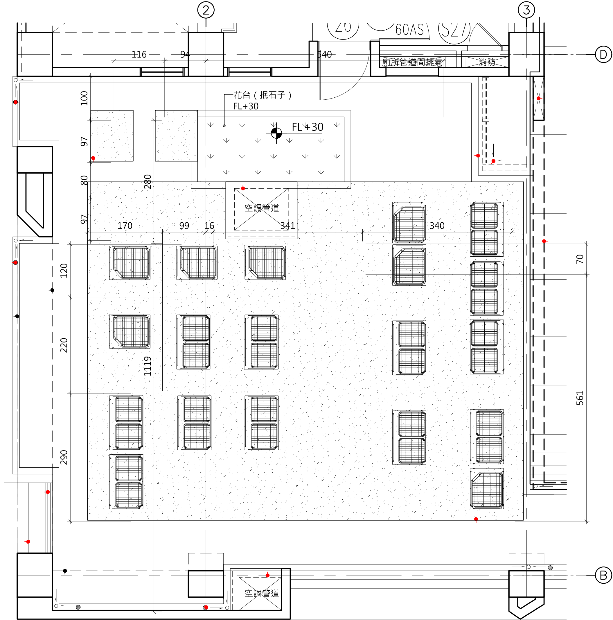
1 屋頂平台平面圖 A1 S:1/50 A3 S:1/100
