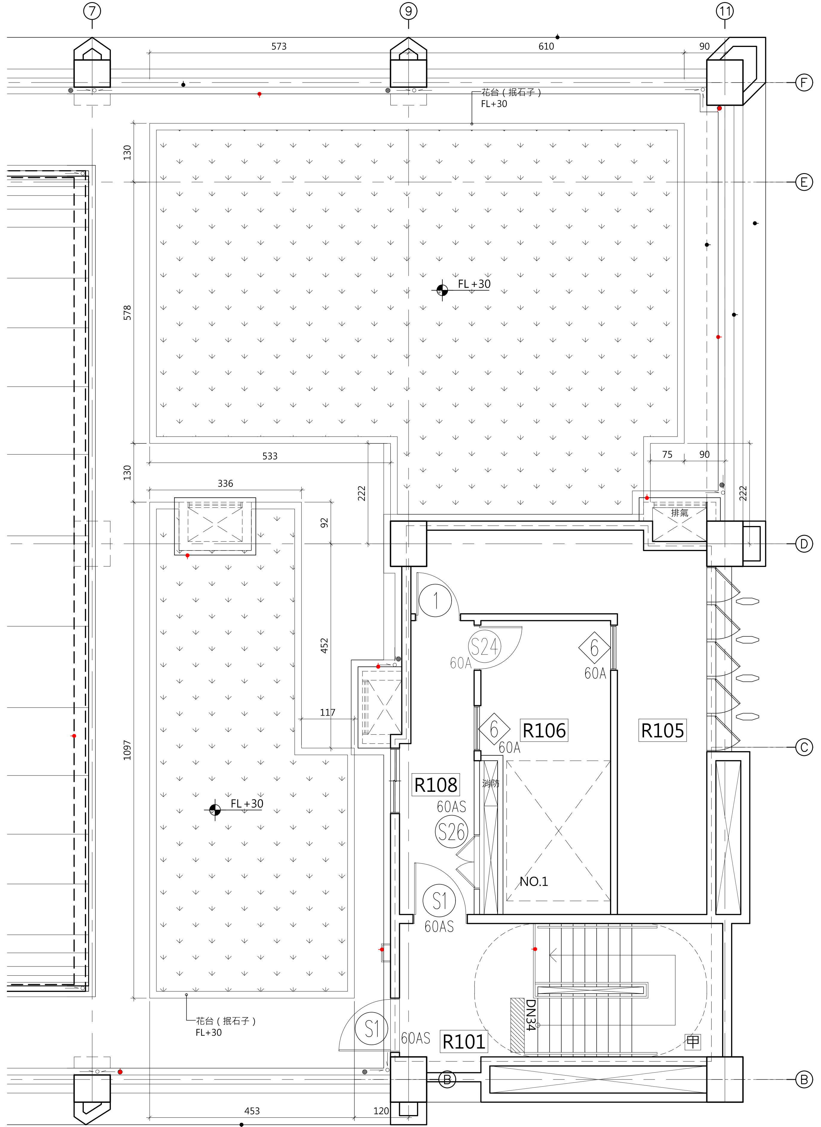
2 屋頂平台平面圖 A1 S:1/50 A3 S:1/100
