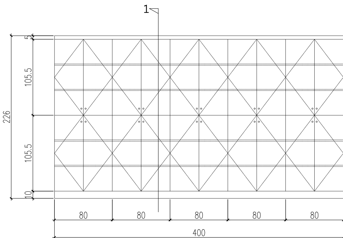
3-2 高櫃立面圖
