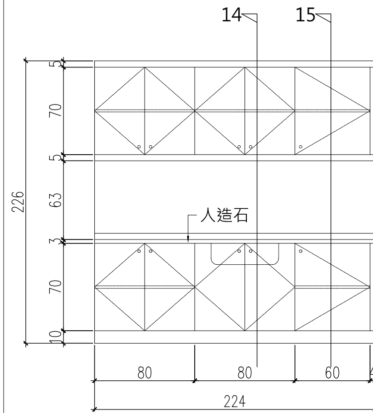
3-6 水槽矮吊櫃立面圖
