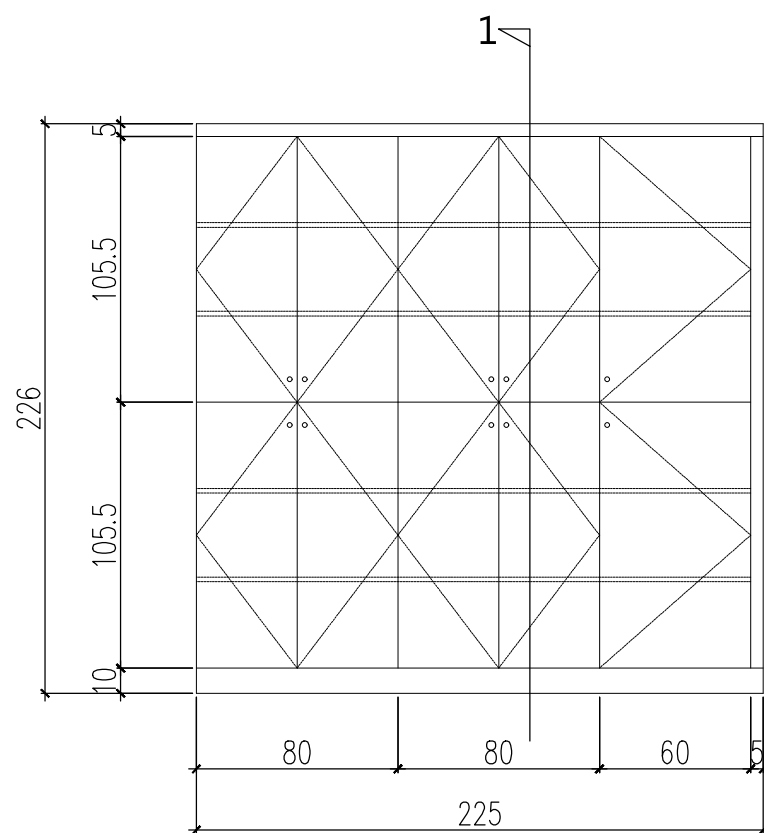
3-3 高櫃立面圖
