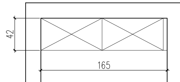
3-4 高櫃平面圖
