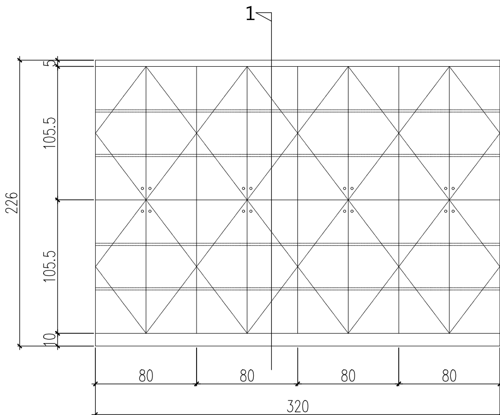
3-5 高櫃立面圖
