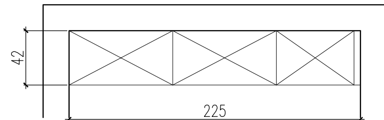
3-3 高櫃平面圖
