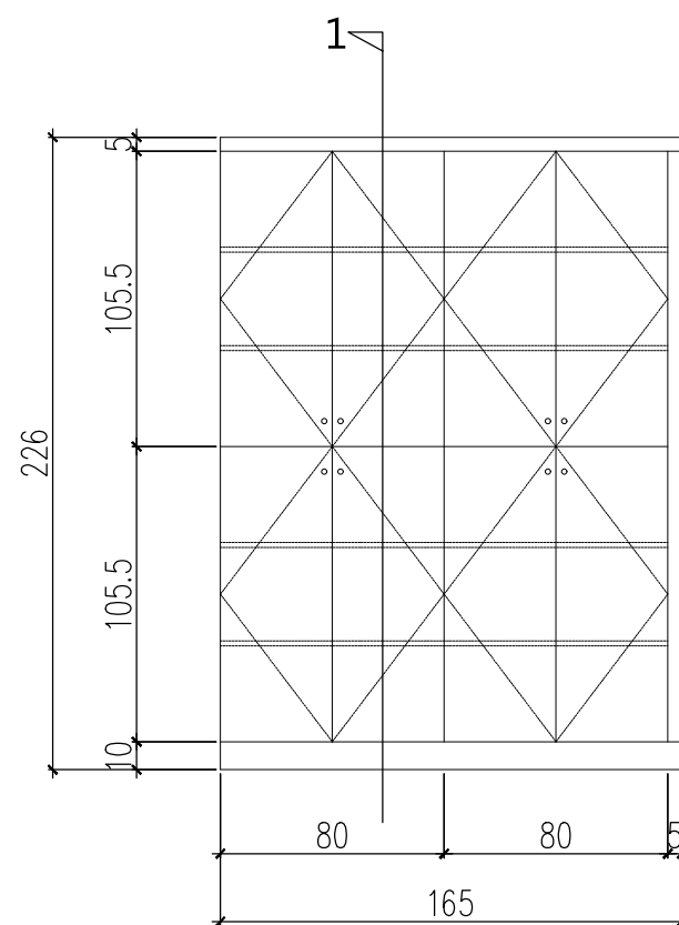
3-4 高櫃立面圖
