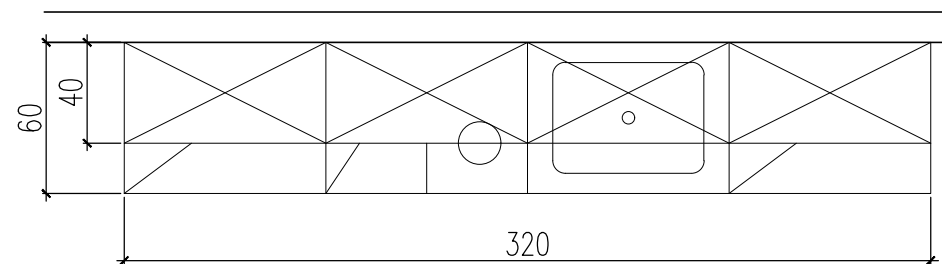
3-8 水槽矮吊櫃平面圖
