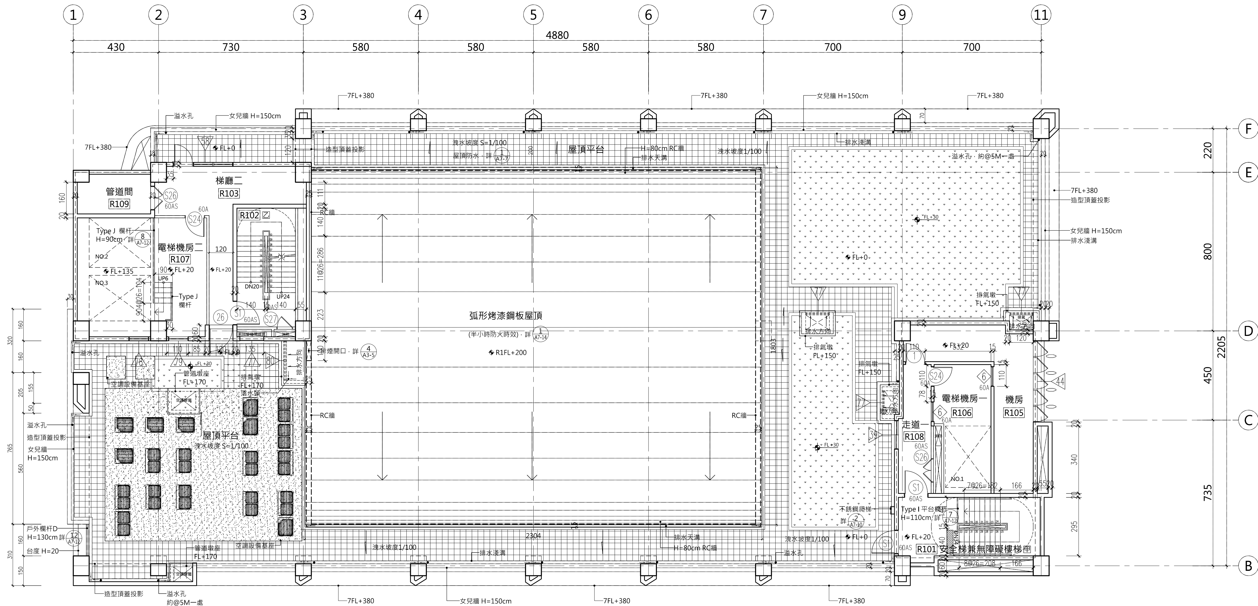
1 屋突一層平面圖
