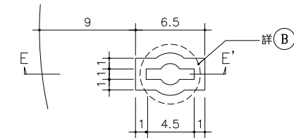
(A) 人孔蓋提舉孔詳圖 Scale: 1/5
