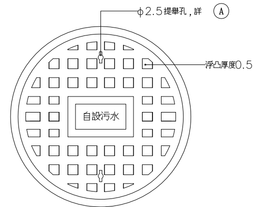
人孔蓋正面圖
