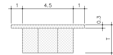
(B) 瓶蓋式橡皮墊物剖面圖 Scale: 1/2
