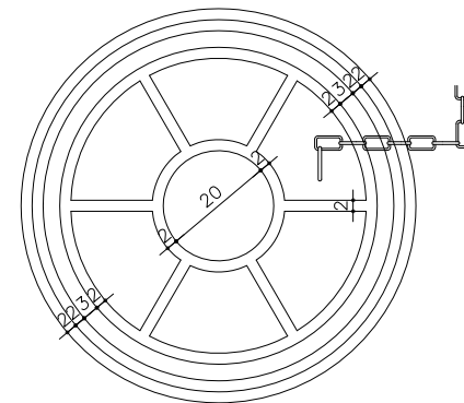
人孔蓋背面圖
