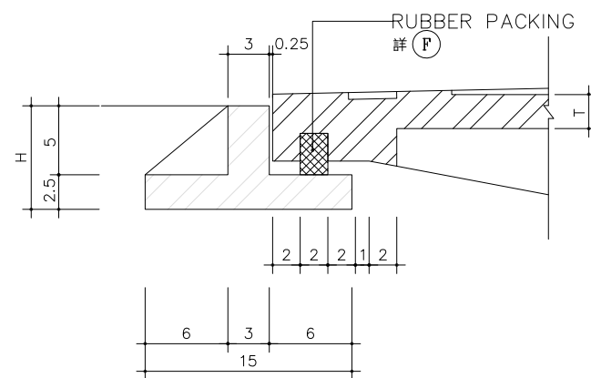
(C) 人孔框蓋接合詳圖 Scale: 1/5
