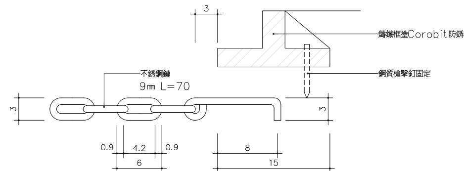
(E) 不銹鋼鏈詳圖 Scale: 1/5
