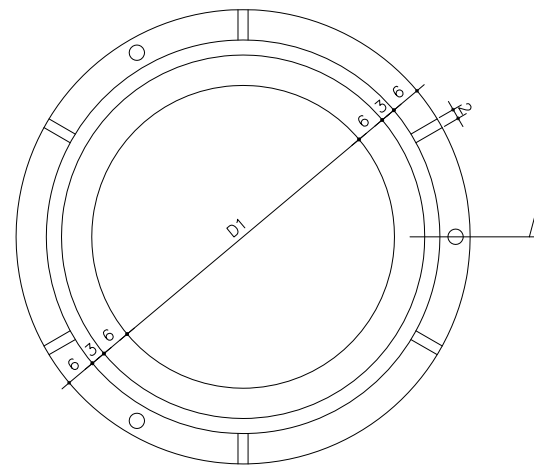
人孔框平面圖
