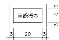
人孔蓋標誌詳圖
