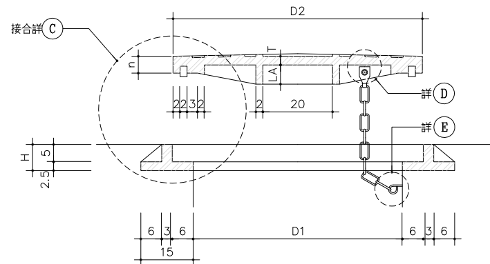
人孔框蓋剖面圖
