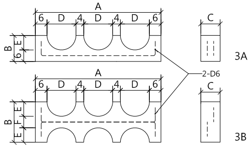
混凝土管路隔離板詳圖
