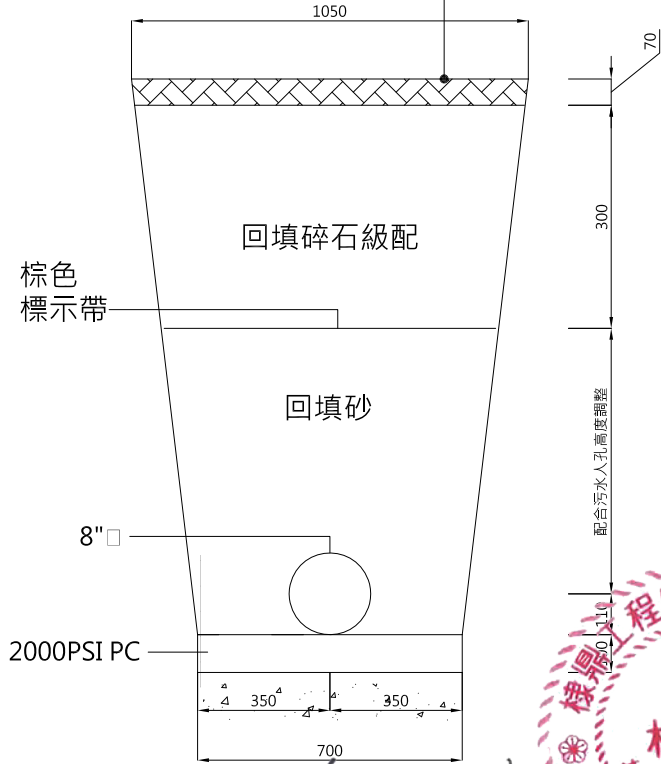
AC或原地坪材質還原
