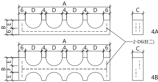
混凝土管路隔離板詳圖
