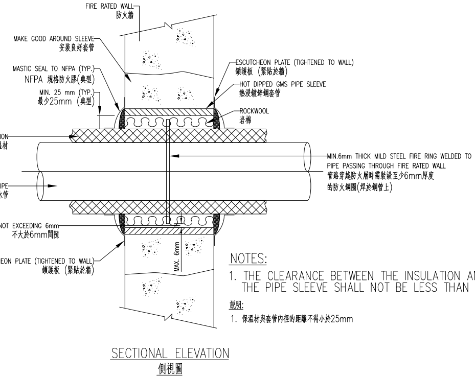
水管穿越防火牆施工詳圖
