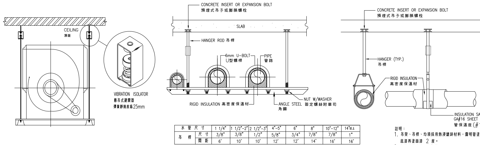
吊裝式風機安裝詳圖
