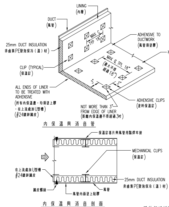
風管保溫詳圖
