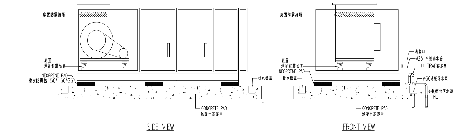
落地式空調箱安裝詳圖
