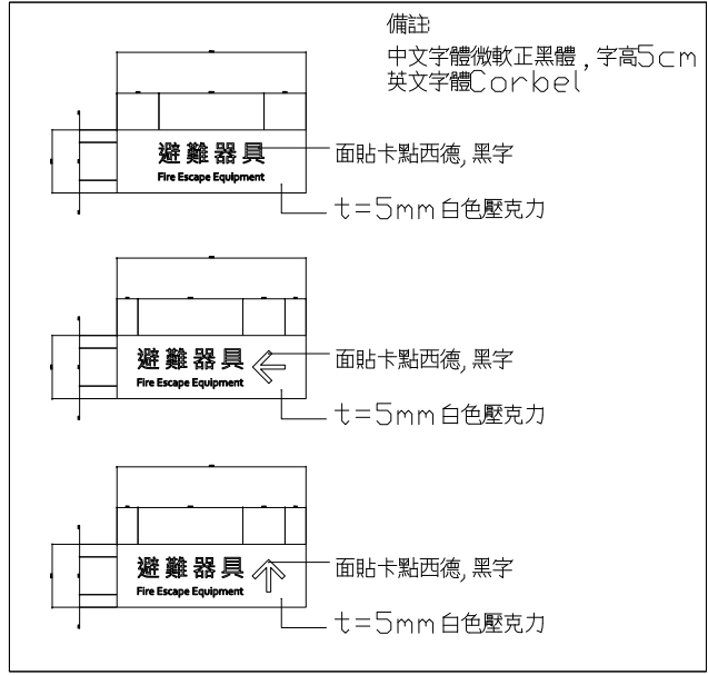
6 避難器具標示牌詳圖 SCALE: 1:10 UNIT: mm
