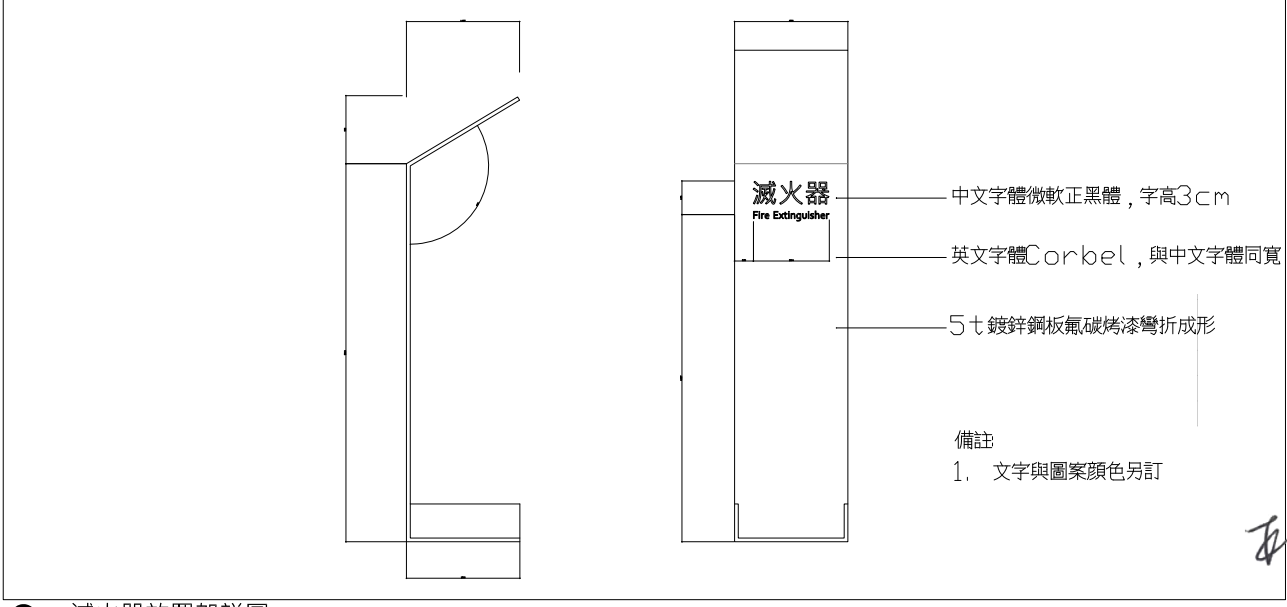
8 滅火器放置架詳圖 SCALE: 1:5 UNIT: mm
