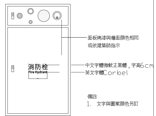
2 消防栓箱立面圖
