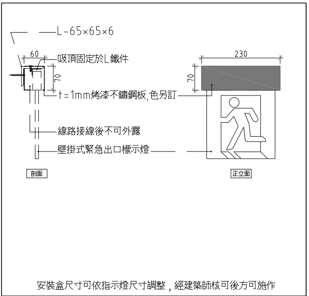
2 消防指示燈安裝盒 Type A SCALE: 1:10 UNIT: mm
