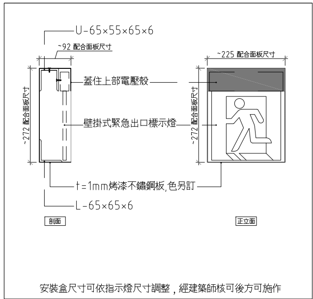
3 消防指示燈安裝盒 Type B SCALE: 1:10 UNIT: mm
