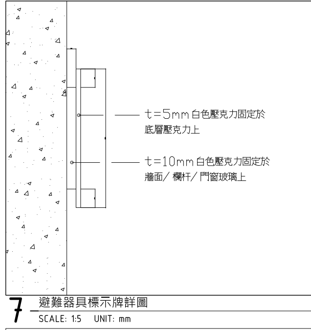
7 避難器具標示牌詳圖 SCALE: 1:5 UNIT: mm
