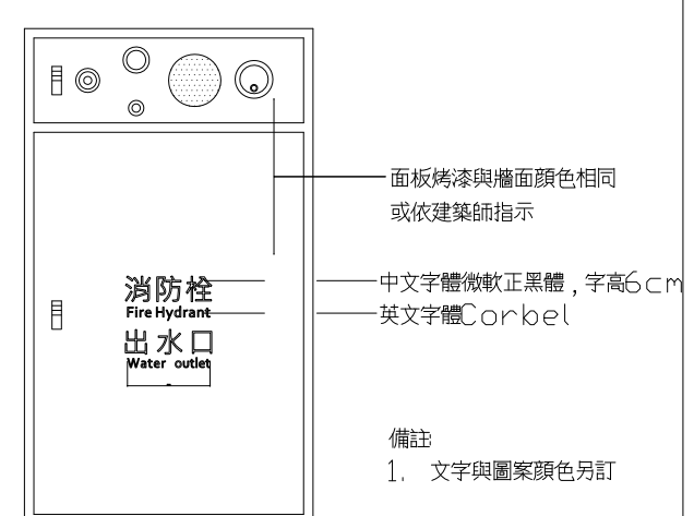
1 綜合消防栓箱立面圖
