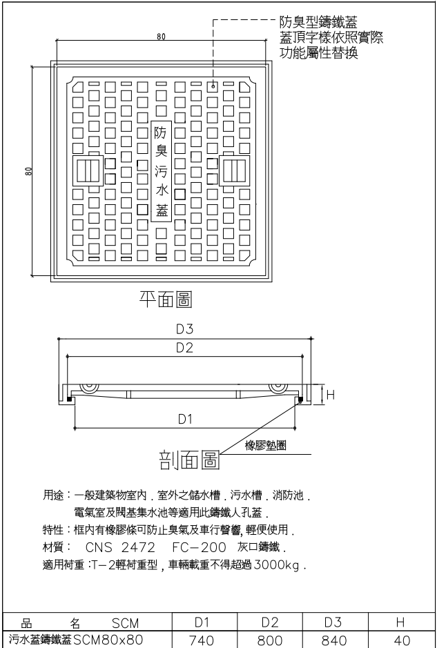
2 防臭型方蓋方框鑄鐵人孔蓋詳圖 SCALE: 1:10 UNIT: mm
