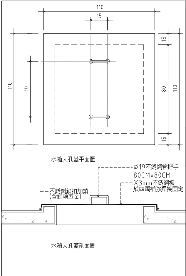
1 生活水箱 人孔蓋詳圖 SCALE: 1:5 UNIT: mm
