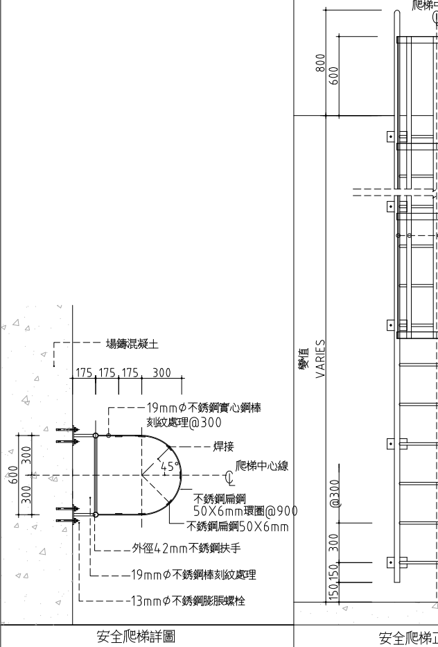
6 安全爬梯詳圖 SCALE: 1:20 UNIT: mm
