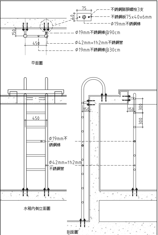
3 生活水箱、泳池水箱 內、外不鏽鋼爬梯詳圖 SCALE: 1:20 UNIT: mm
