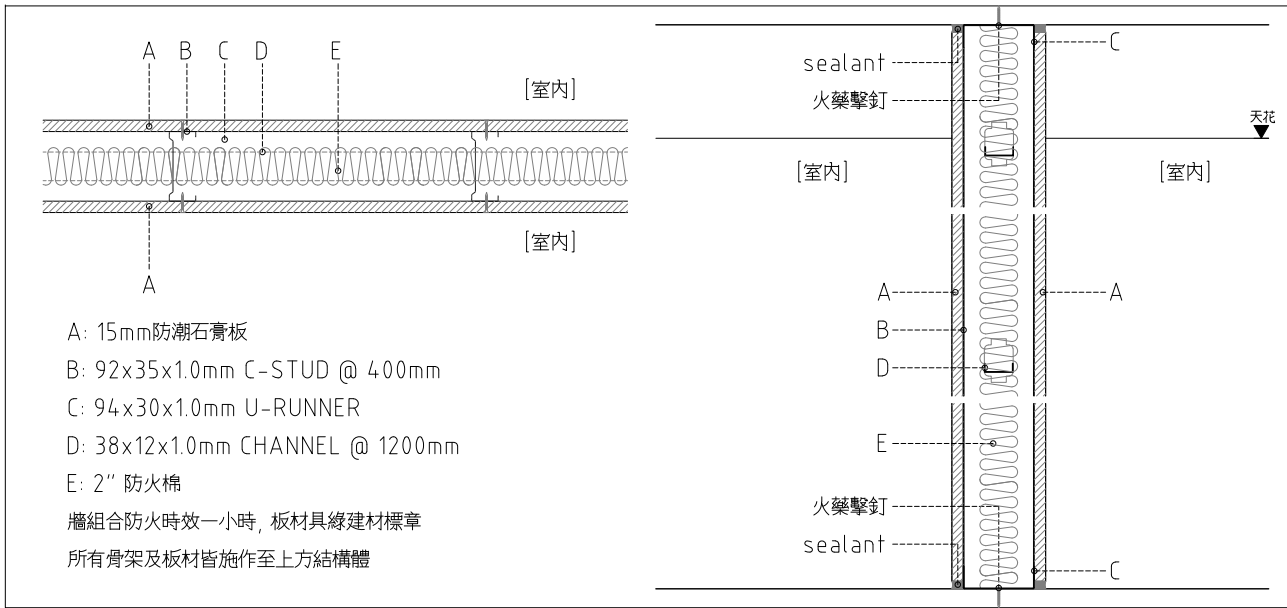
1 TYPE A: 一般乾式內牆 SCALE: 1:5 UNIT: mm
