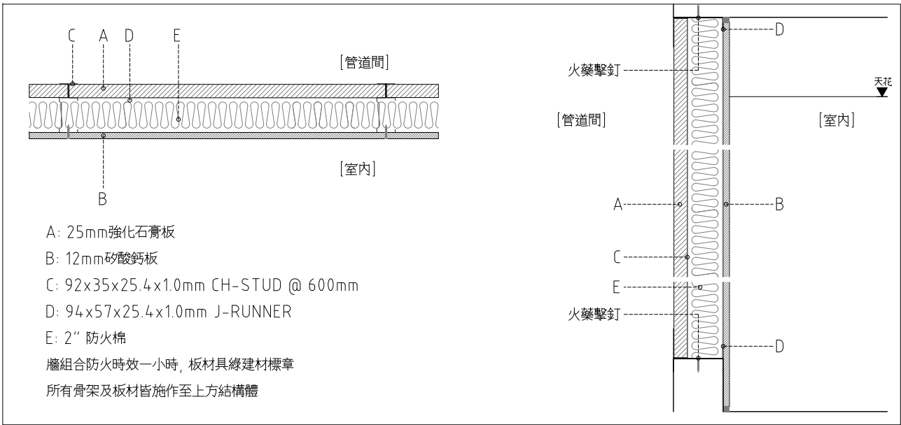
2 TYPE B: 管道間乾式內牆 SCALE: 1:5 UNIT: mm
