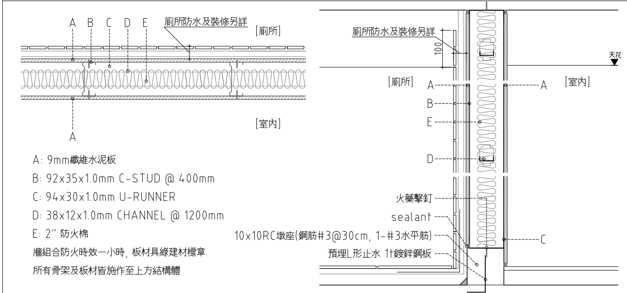
3 TYPE C: 廁所乾式內牆 SCALE: 1:5 UNIT: mm
