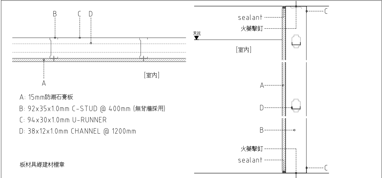
4 TYPE D: 乾式內牆單面封板 SCALE: 1:5 UNIT: mm
