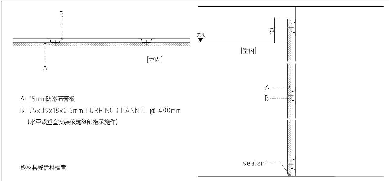
5 TYPE E: 乾式裝修封板 SCALE: 1:5 UNIT: mm
