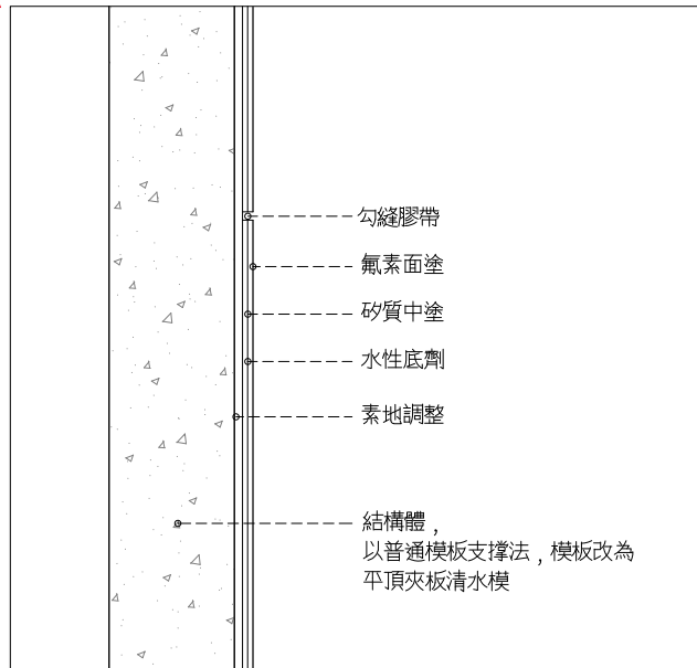
外牆夾板模板後製清水模工法 詳圖
