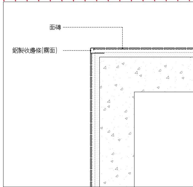
3 廁所面磚轉角收邊條詳圖
