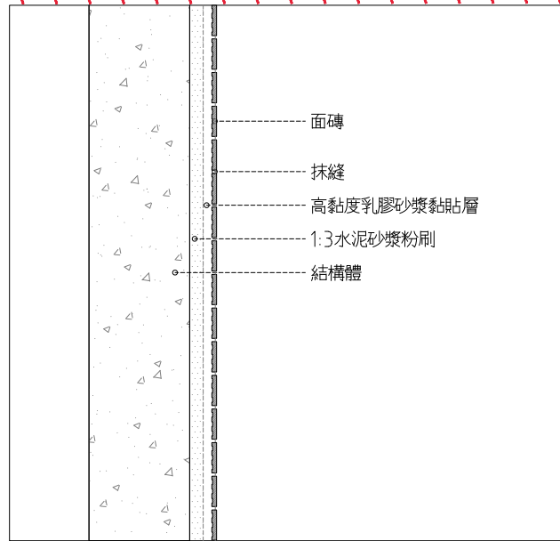
面磚牆面 詳圖
