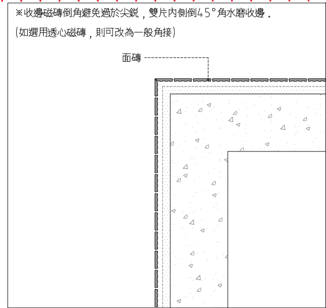
一般空間面磚轉角收邊詳圖
