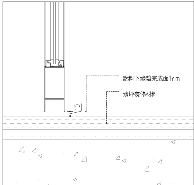
6 室內門 下部詳圖 SCALE: 1:2.5 UNIT: mm
