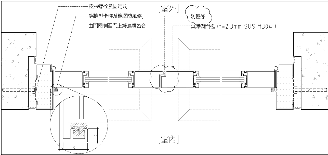
7 對外落地門 平面詳圖 SCALE: 1:2.5 UNIT: mm
