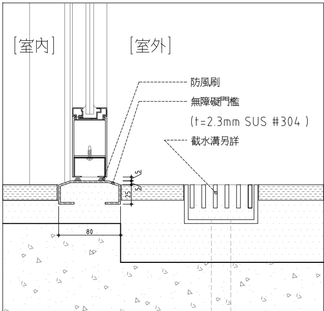
4 對外落地門 門檻詳圖 SCALE: 1:2.5 UNIT: mm
