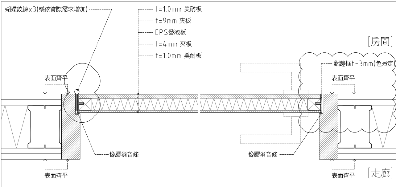
5 EPS美耐板門 (TYPE A) 細部詳圖 SCALE: 1:2.5 UNIT: mm
