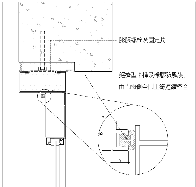
3 室內門 頂部詳圖 SCALE: 1:2.5 UNIT: mm
