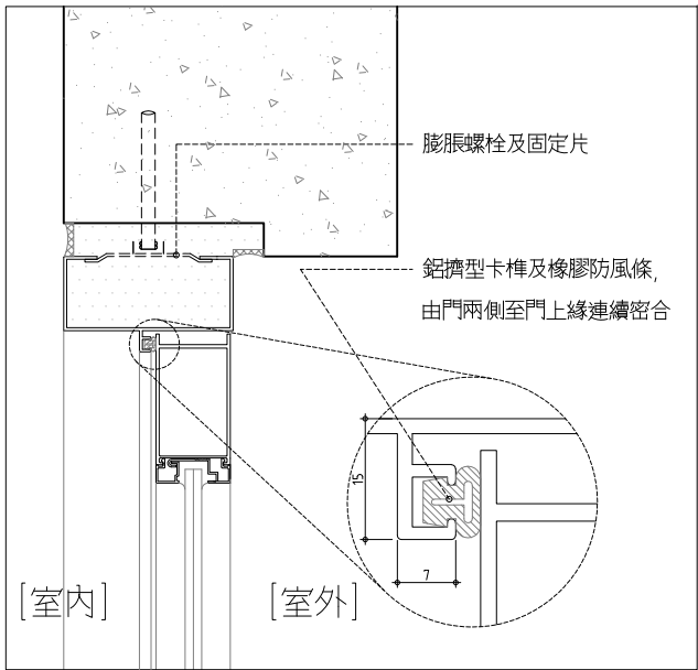
1 對外落地門 頂部詳圖 SCALE: 1:2.5 UNIT: mm
