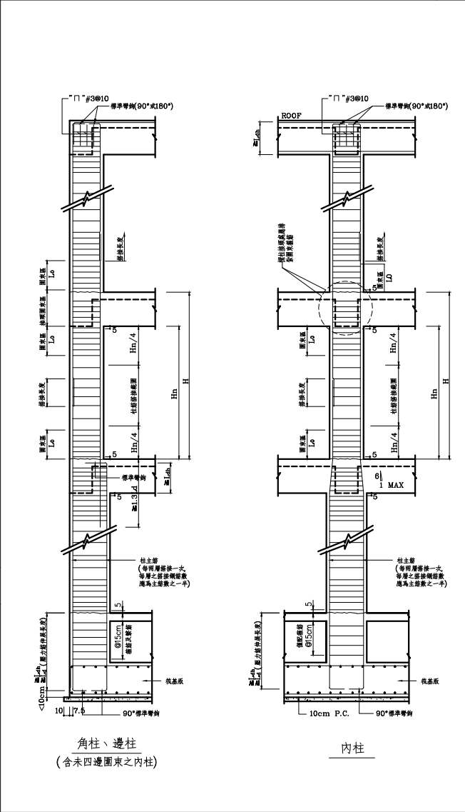
柱配筋標準圖
