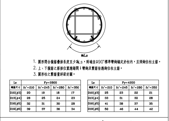
圓柱閉合箍筋示意圖 (外箍以疊接加標準彎鉤固定接合時)
