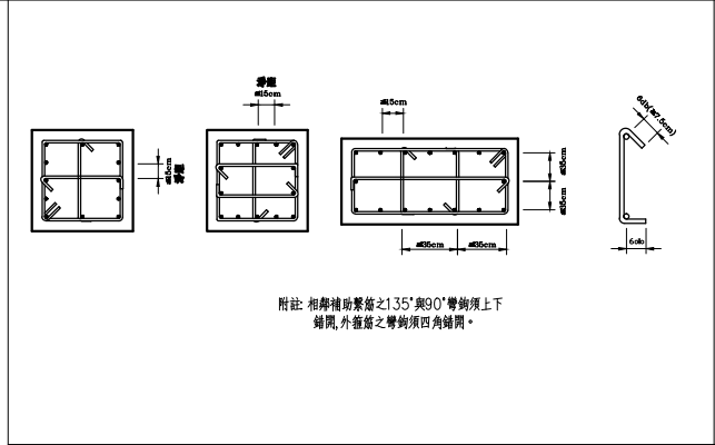
矩形柱箍筋示意圖
