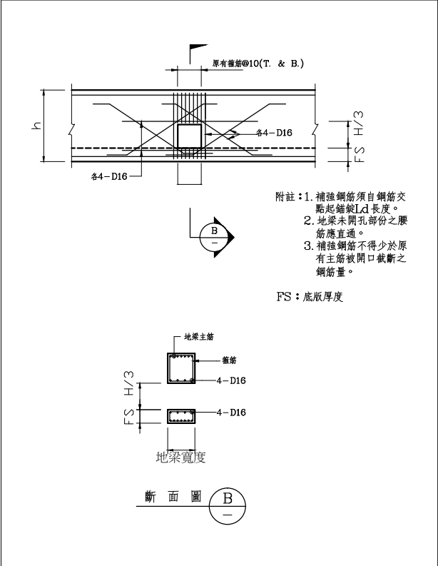
地梁穿孔補強詳圖
