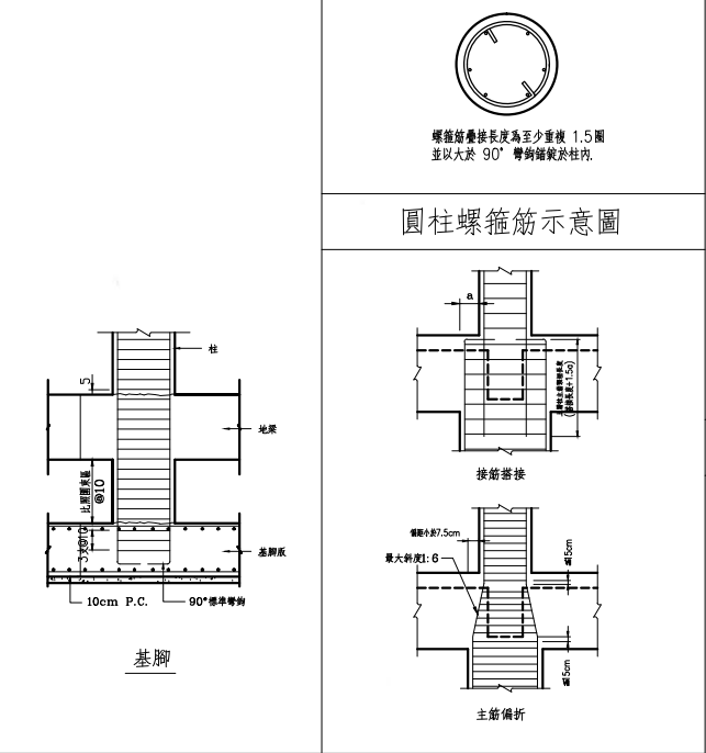
圓柱螺箍筋示意圖
