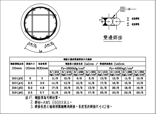
圓柱閉合箍筋示意圖 (外箍以焊接接合時)
