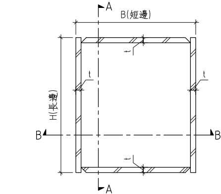
箱型柱現場續接詳圖 箱型柱尺寸標示：Box-HxBxtxt
