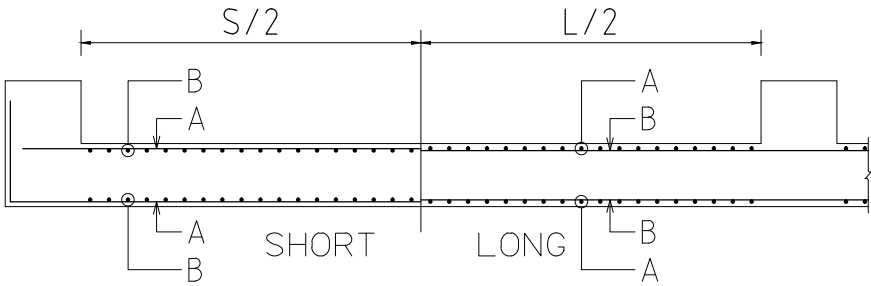
FS版配筋圖
