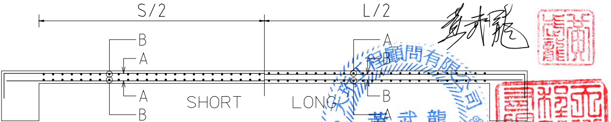
B1F~1F BS版,S版配筋圖
