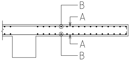
懸臂版配筋圖
