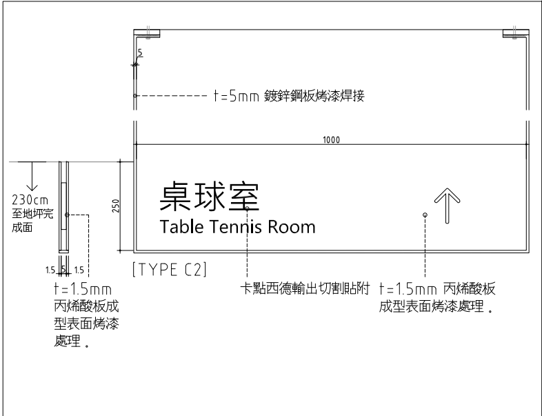
03 指標 TYPE S: 懸吊式標示牌 SCALE: UNIT: mm
