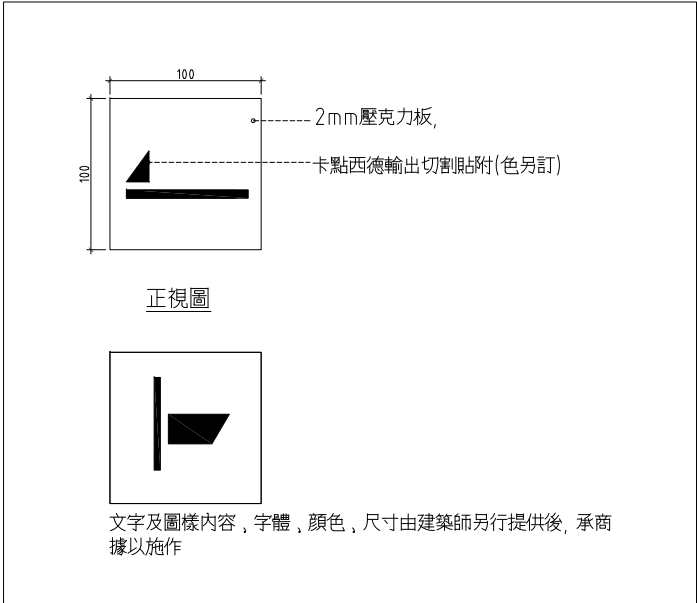
04 指標 TYPE E: 廁所標示(貼壁式) SCALE: UNIT: mm
