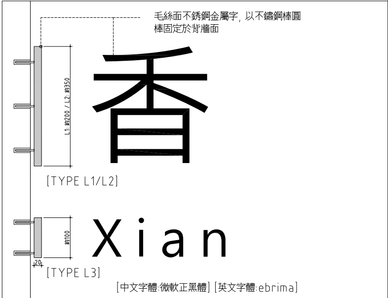
06 指標TYPE L1/L2/L3: 掛牆式金屬字 SCALE: UNIT: mm
