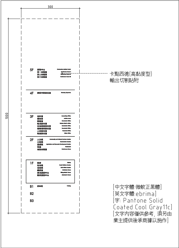
01 指標 TYPE D: 樓層簡介指標 SCALE: UNIT: mm
