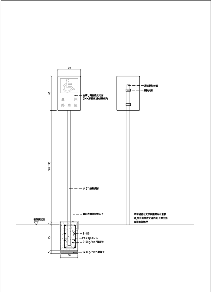
02 指標 TYPE P2: 無障礙專用停車位標示(直立式) SCALE: UNIT: mm
