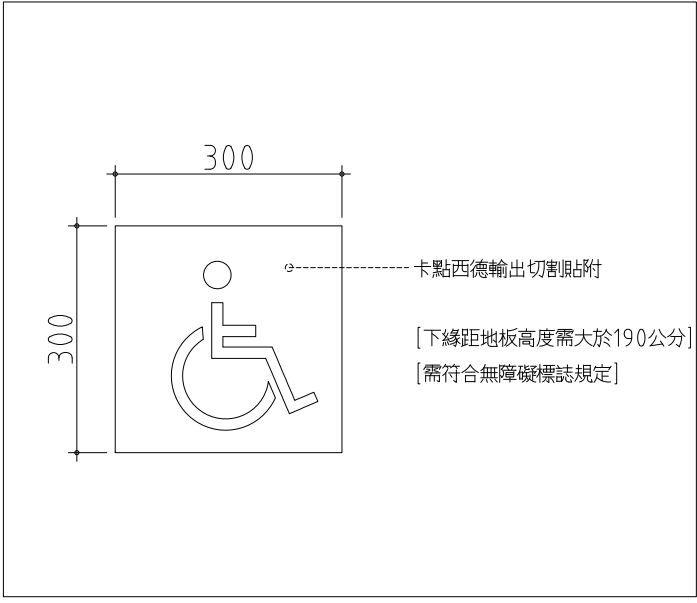
05 指標 TYPE P1: 無障礙專用停車位標示(貼壁式) SCALE: UNIT: mm
