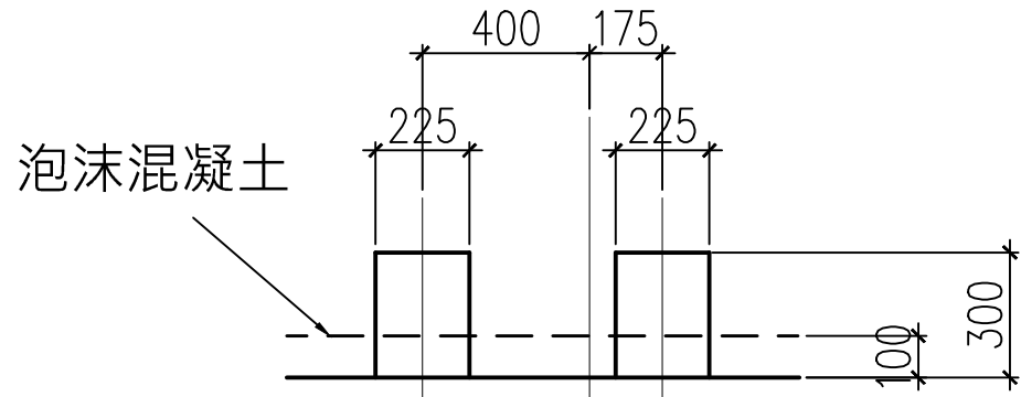
B-B視圖
