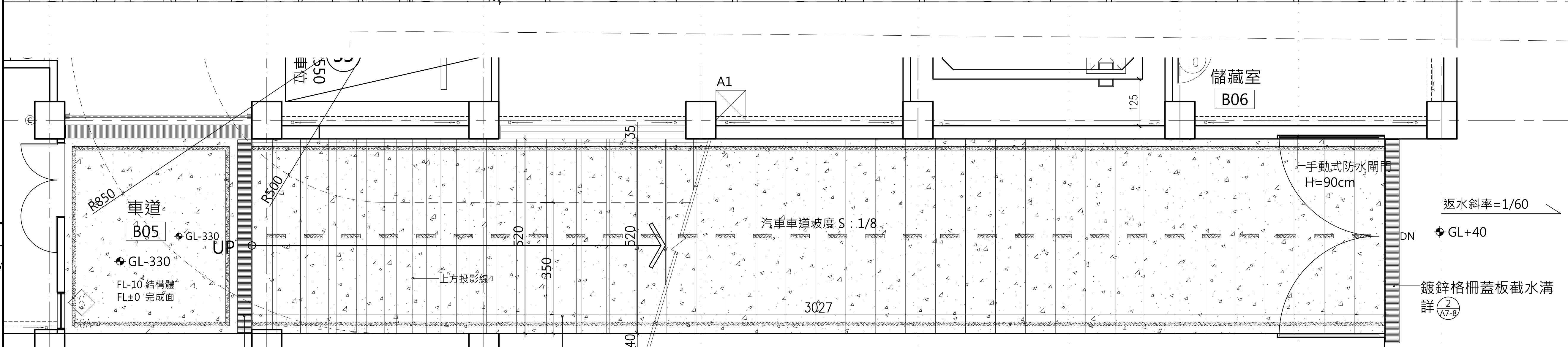
1 車道平面圖 A1 S:1/60 A3 S:1/120
