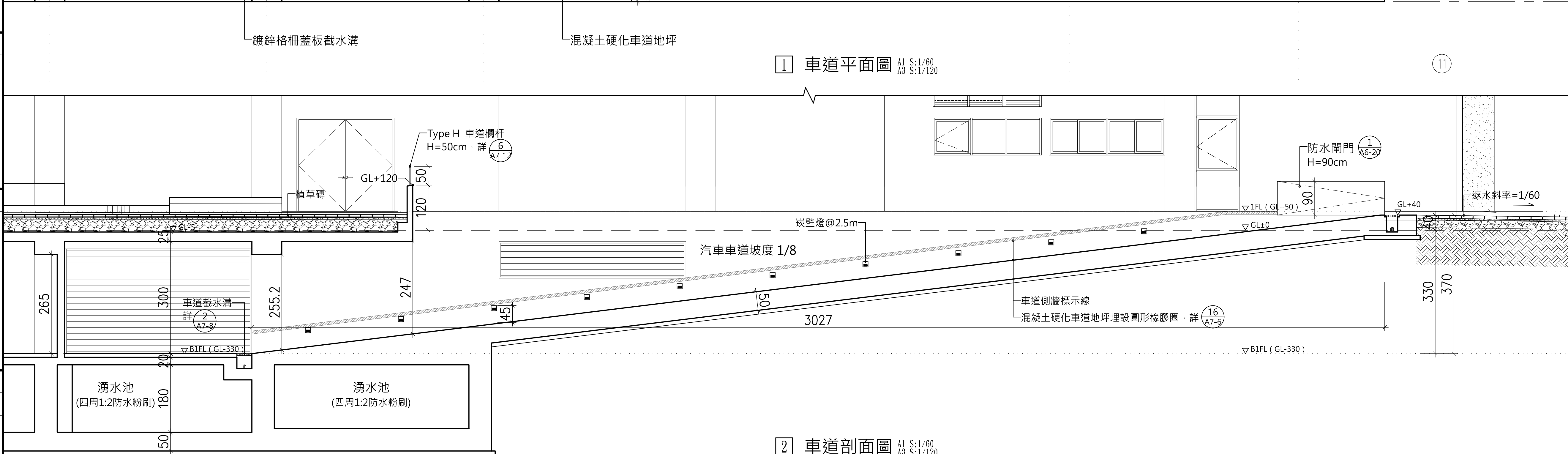
2 車道剖面圖 A1 S:1/60 A3 S:1/120
