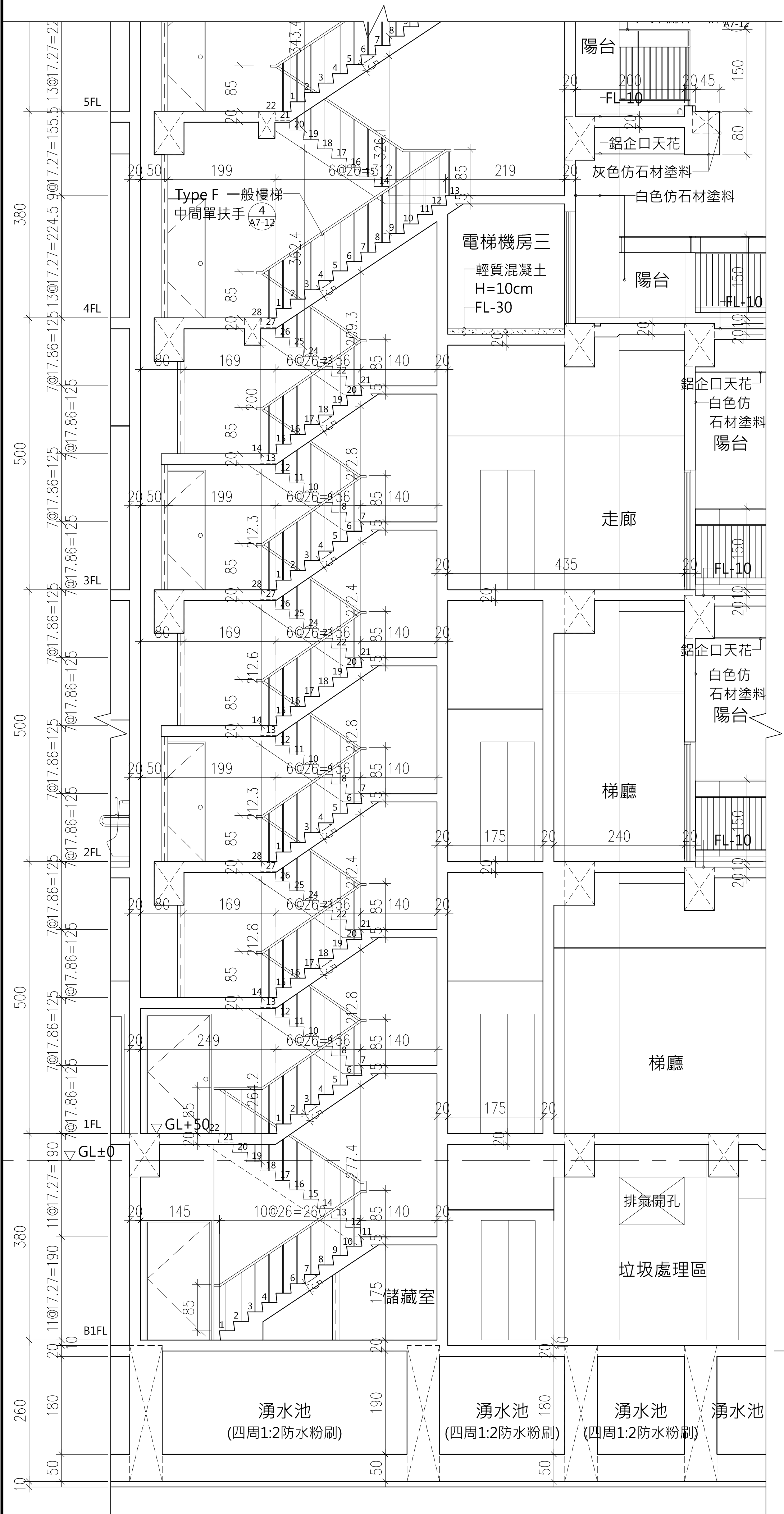
1 乙梯剖面圖
