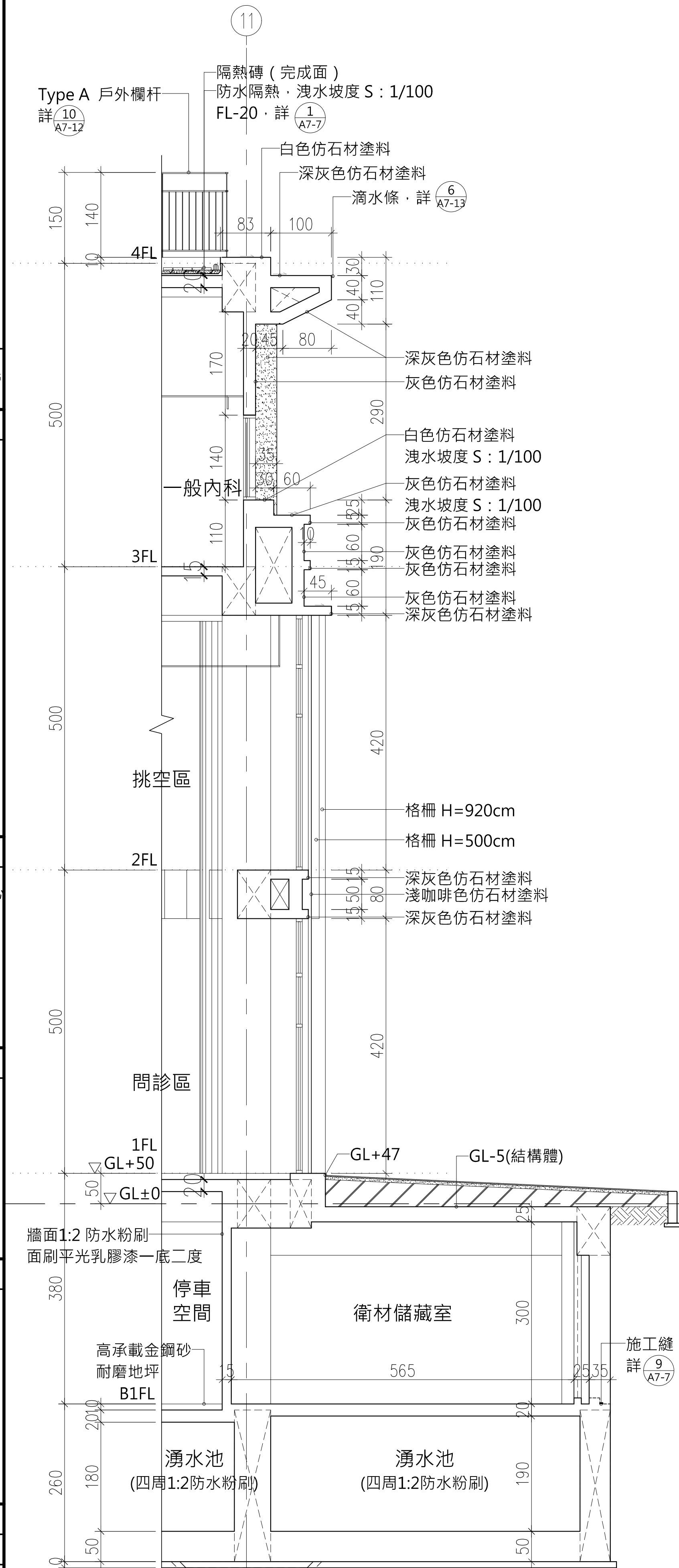
1 外牆剖面圖(11) A1 S:1/50 A3 S:1/100
