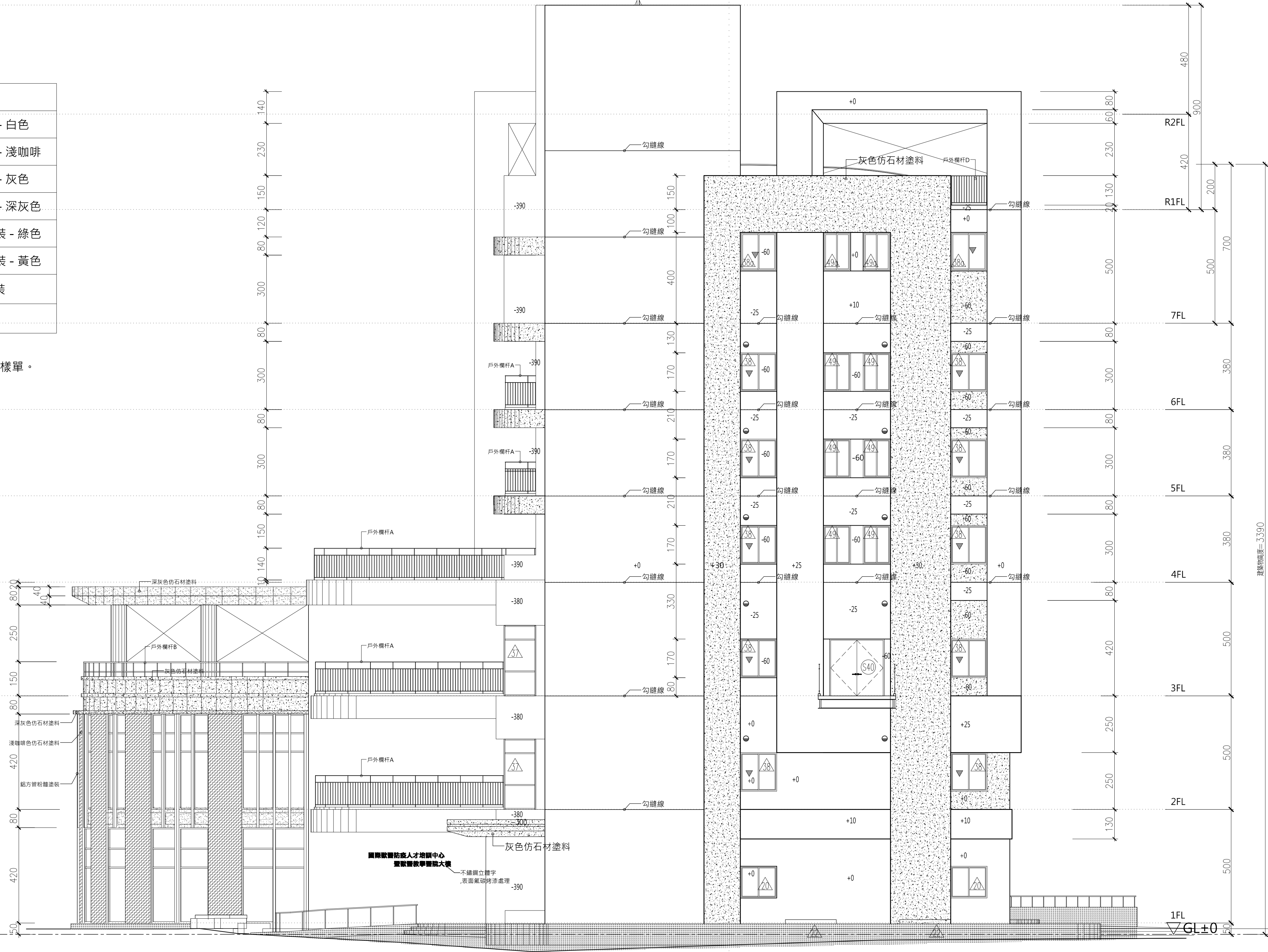
3 西向立面圖 S:A1=1/100 ,A3=1/200
