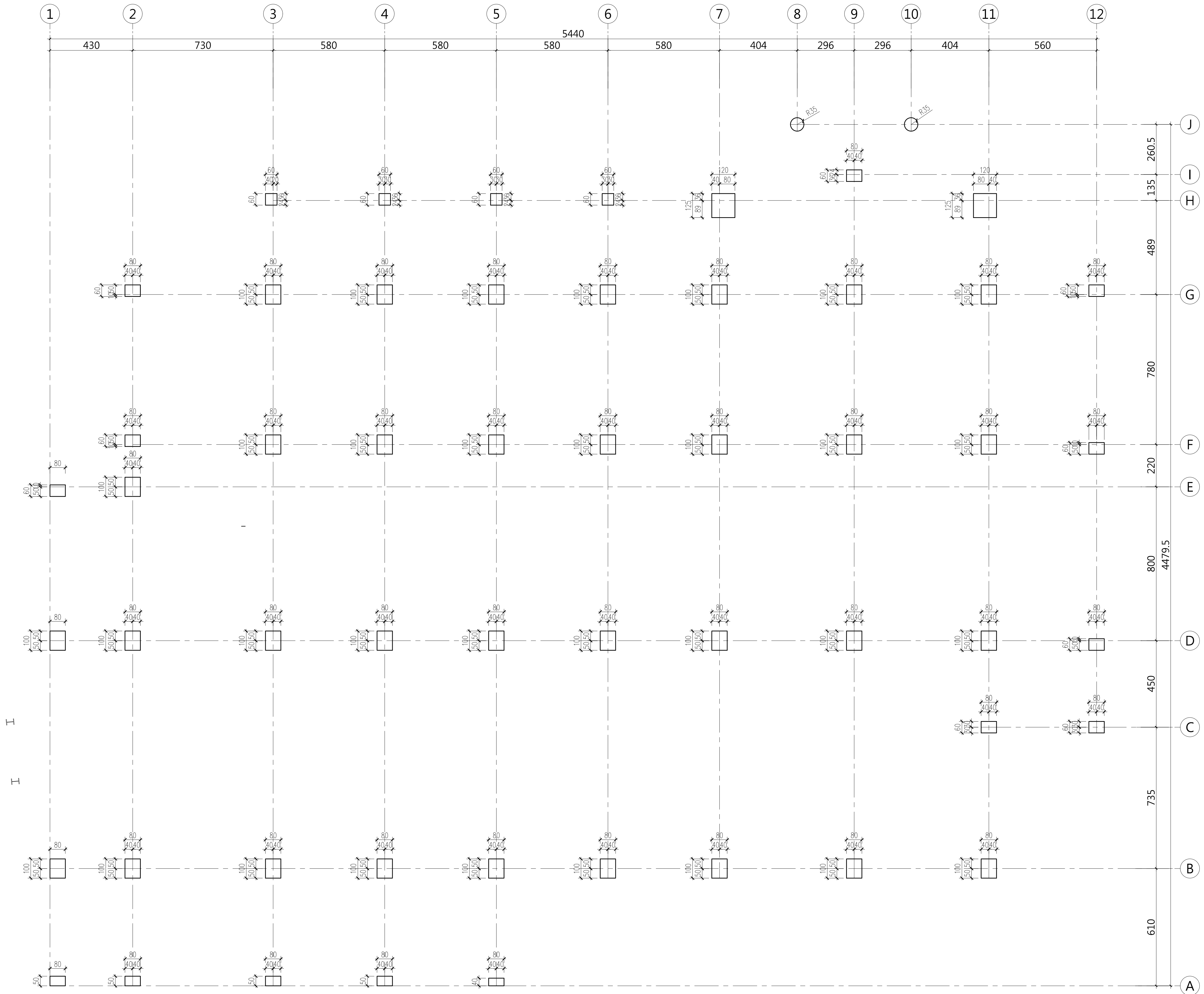
1 地下一層柱位放樣平面圖
