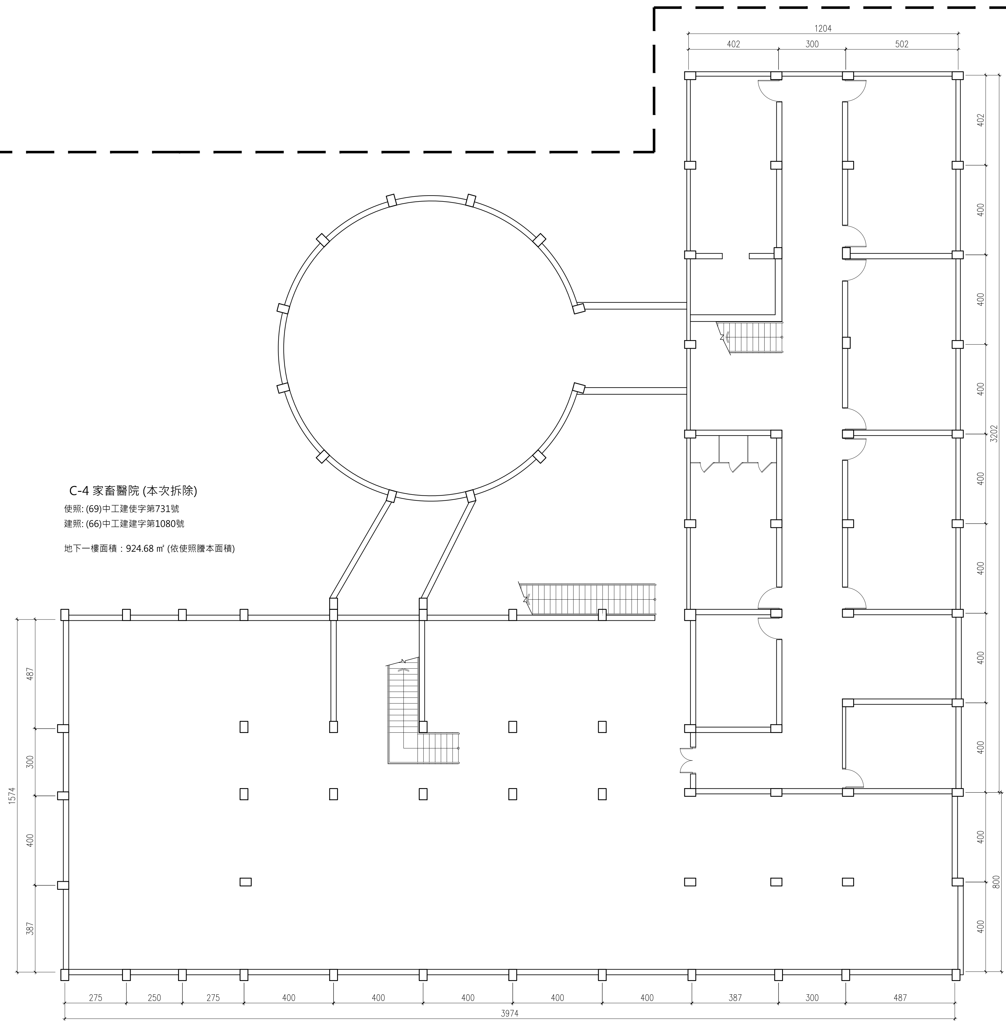
1 地下一層原有建物拆除平面圖
